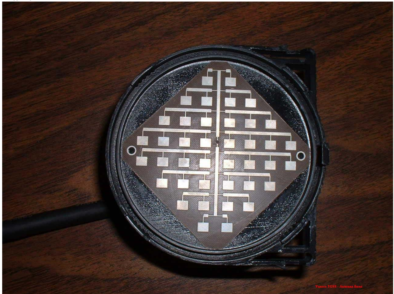
Antenna
