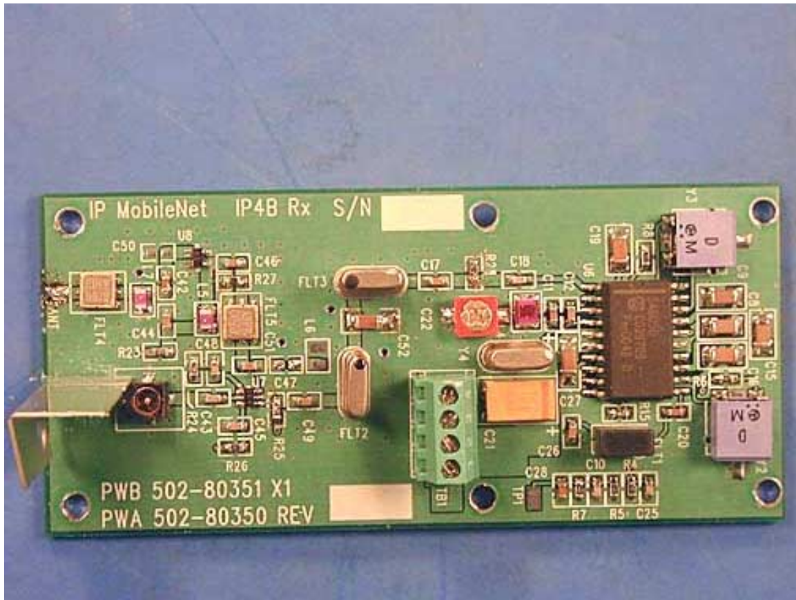
RX PCB Top
