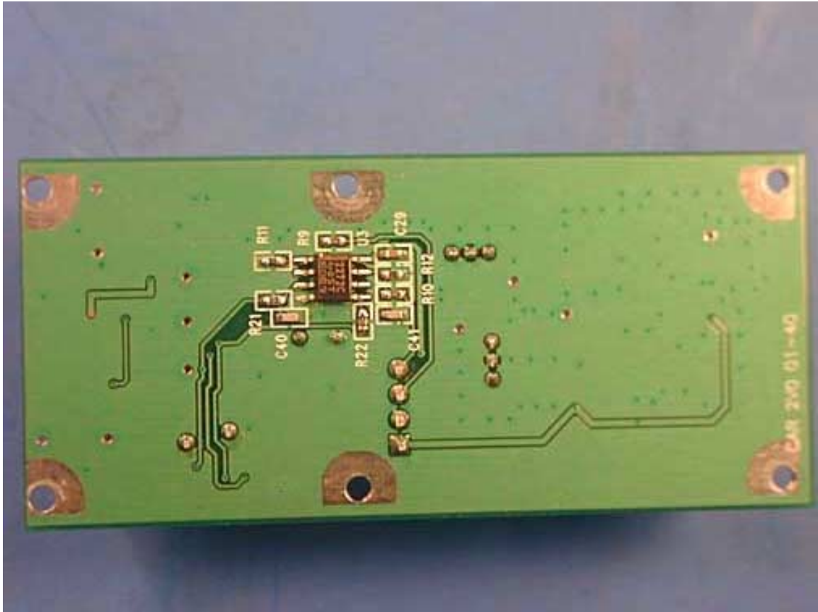
RX PCB Bottom
