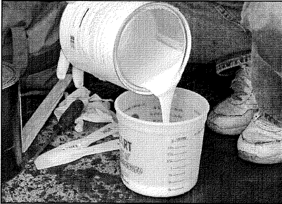
STEP 10 - Pour one quart of Bondo epoxy PART A into a disposable bucket.
