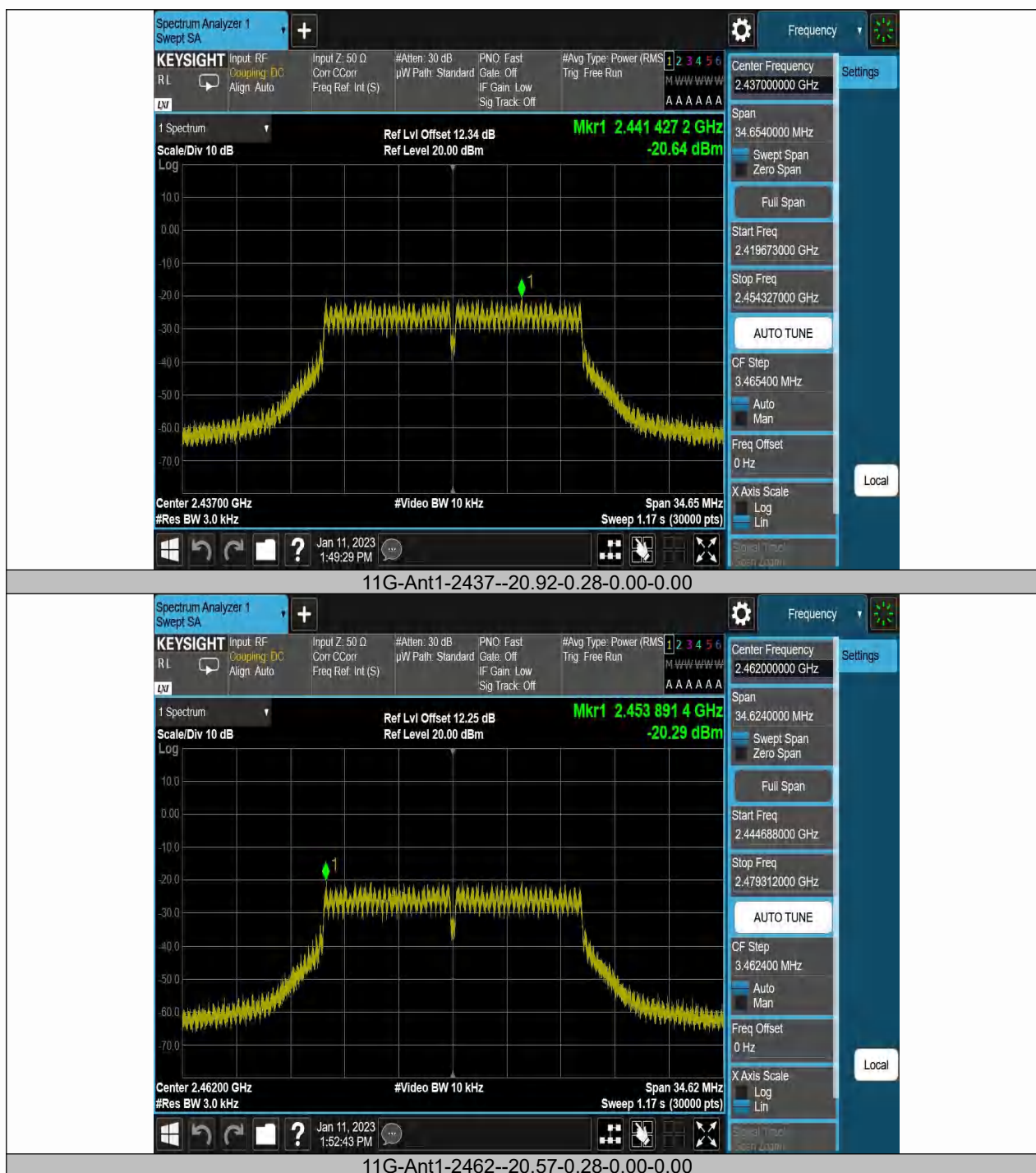
11G-Ant1-2462--20.57-0.28-0.00-0.00
