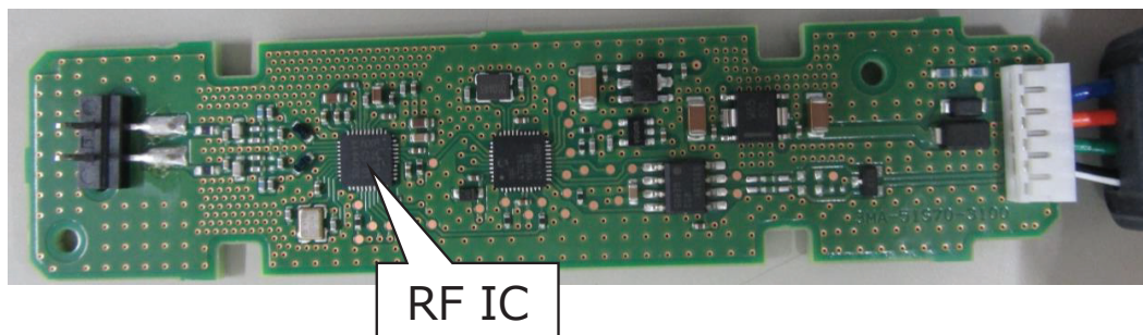
・制御基板 表面 (Control Circuit board -FRONT)
