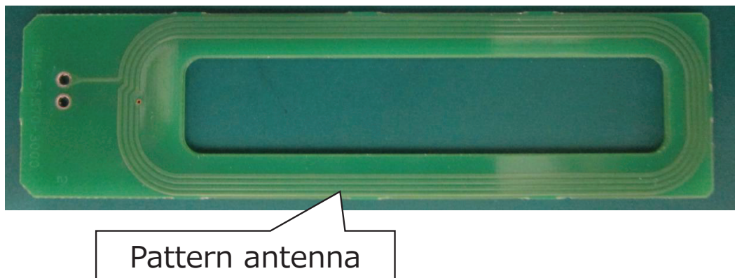
・アンテナ基板 表面 (ANTENNA-FORNT)
