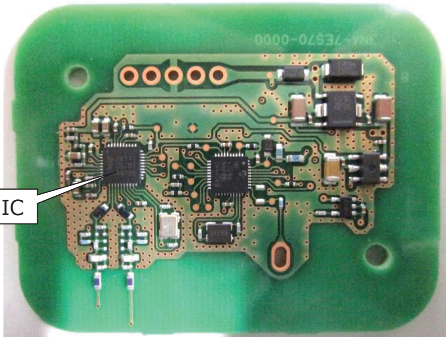
•制御/アンテナ基板 表面 (Control Circuit/ANTENNA board -FRONT)
