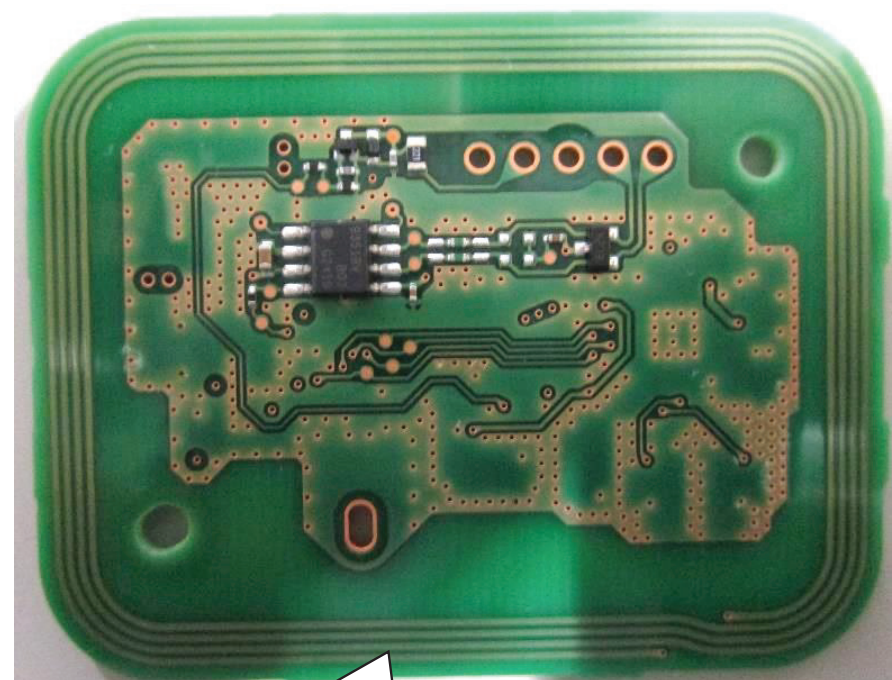
•制御/アンテナ基板 表面 (Control Circuit/ANTENNA board -BACK)
