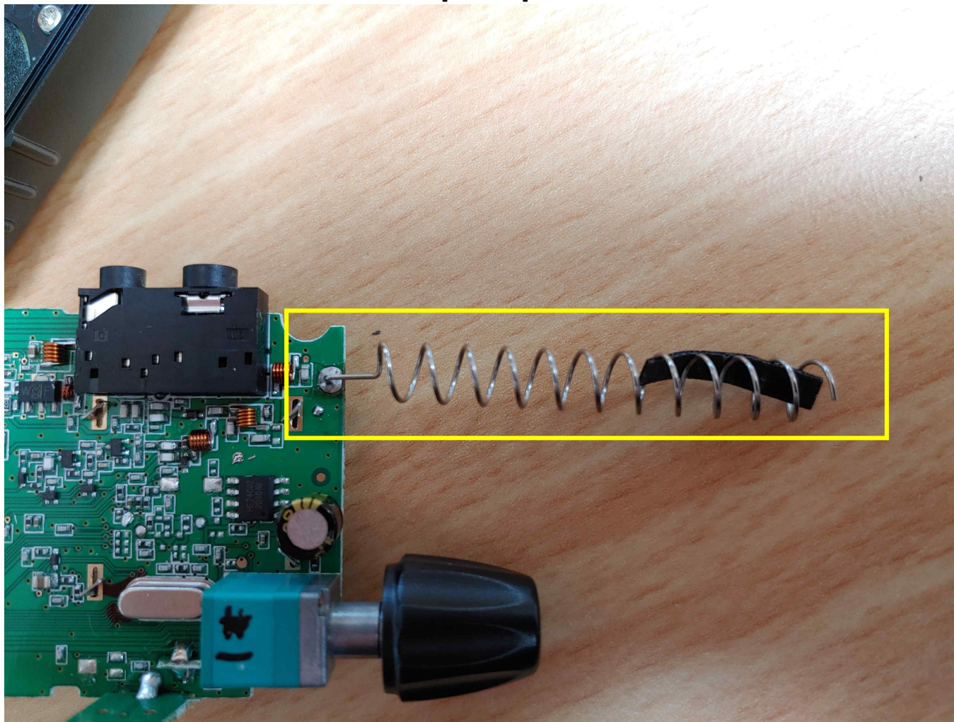
[Antenna]
