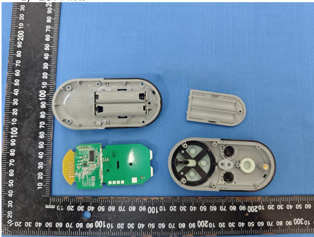
2) EUT Photo
