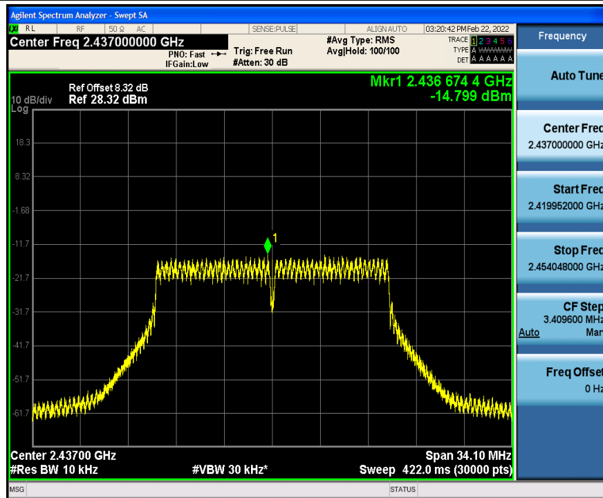
11G_Ant1_2437
