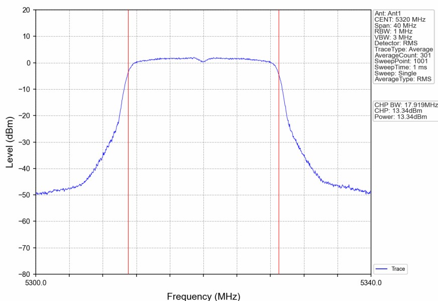
802.11n(HT20)_HCH_5320MHz_Ant1_NTNV
