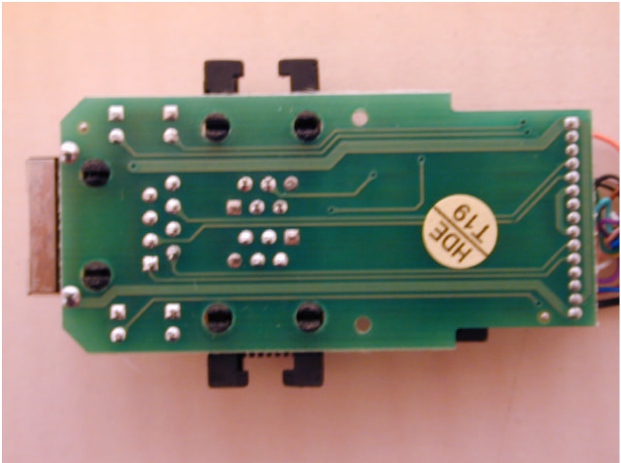
(12) EUT Photo
