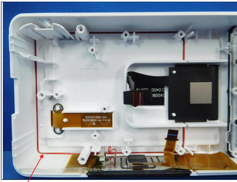
NFC Antenna
