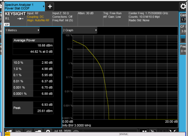
10MHz / 16QAM
