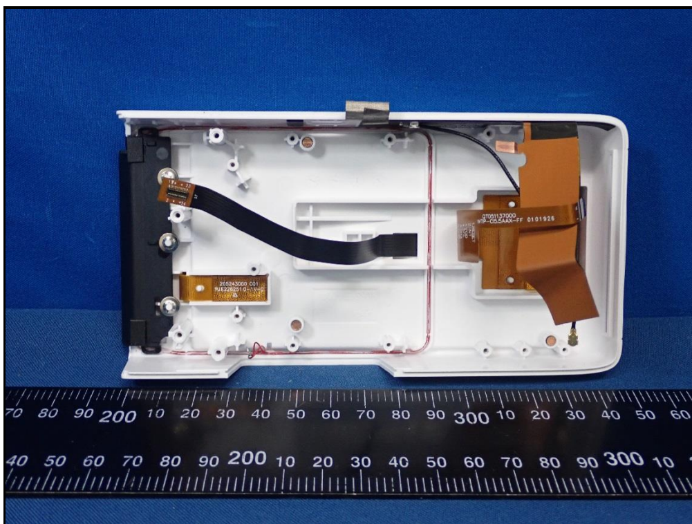
Antenna-NFC
