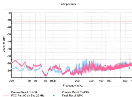
Figure 347: GMSK 16000bps, Ch Width 25kHz, 450.5 MHz, Y
