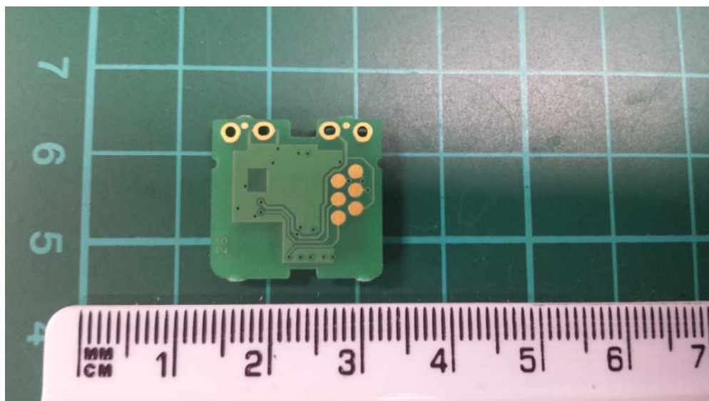
(9) EUT Photo
