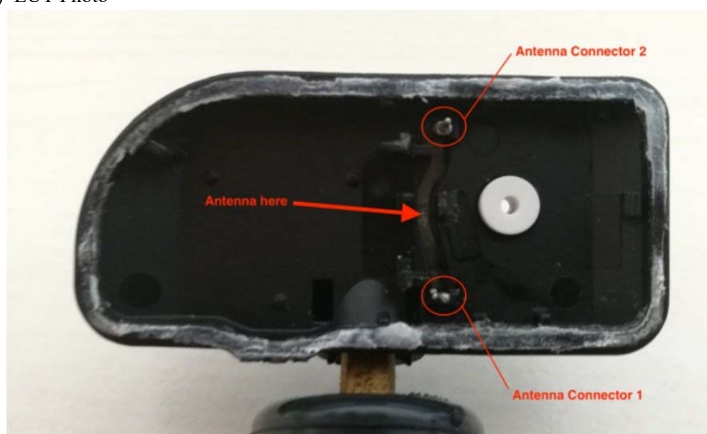
(10) EUT Photo
