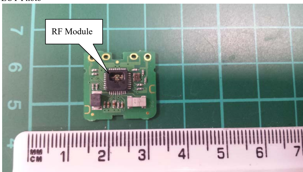
(8) EUT Photo
