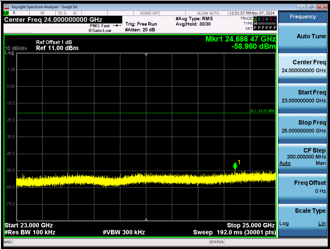
11B-2462-23000~25000-PASS
