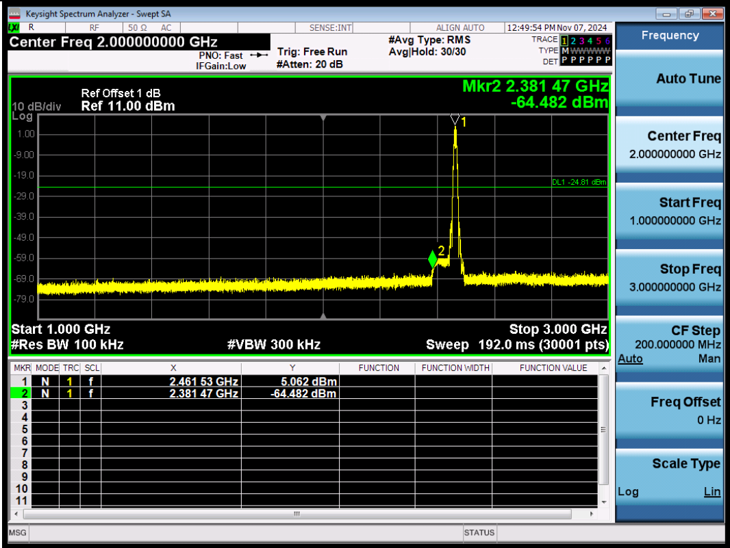
11B-2462-1000~3000-PASS
