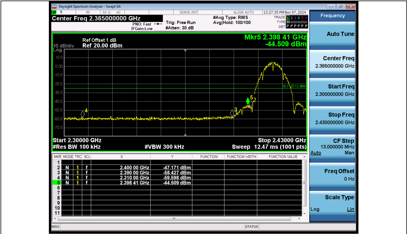
11B-2412-PASS
