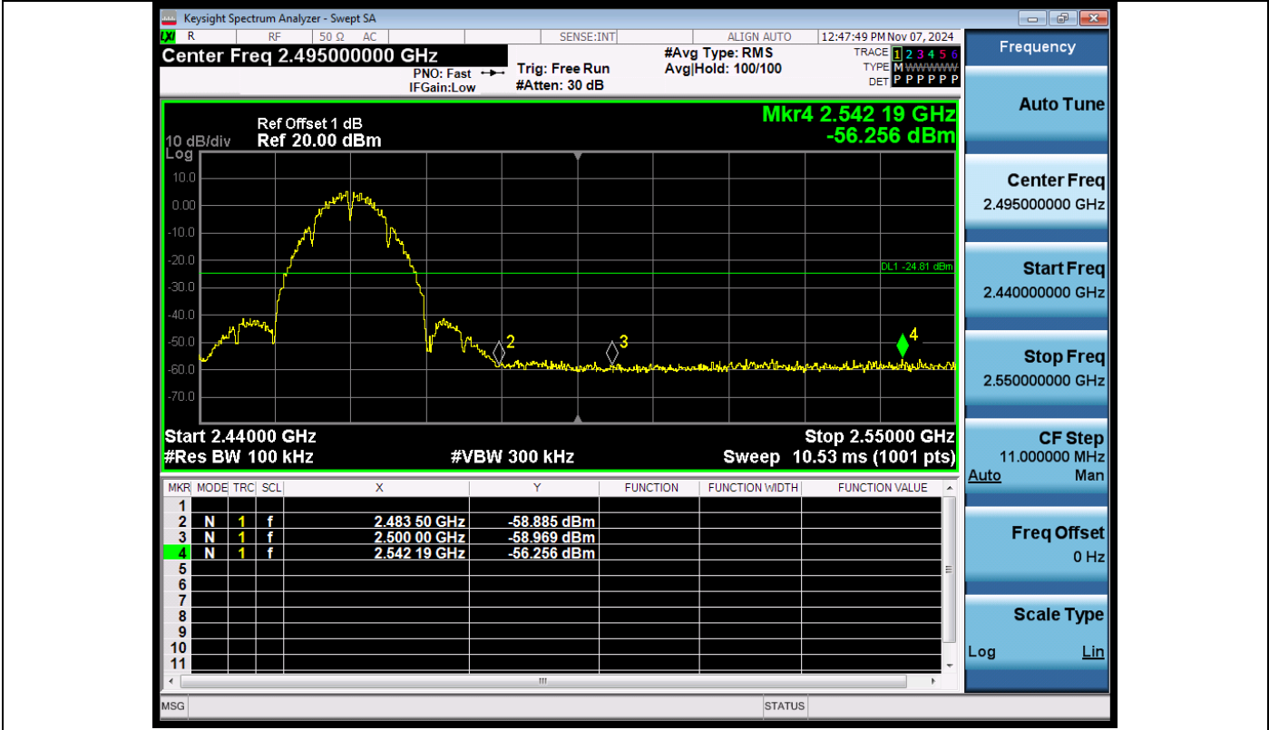
11B-2462-PASS
