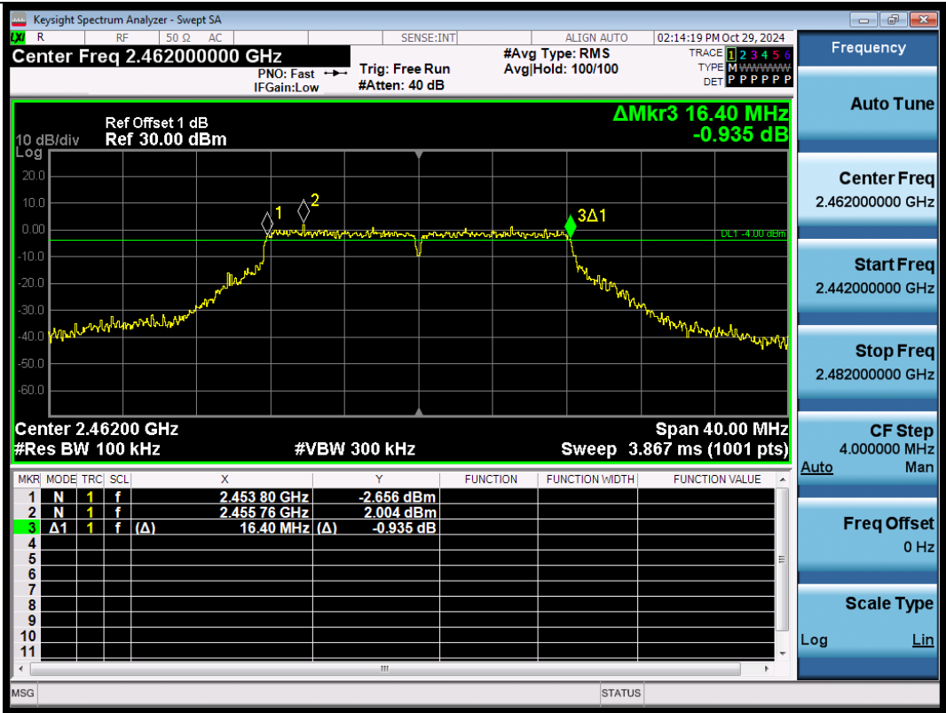
11G-2462-PASS
