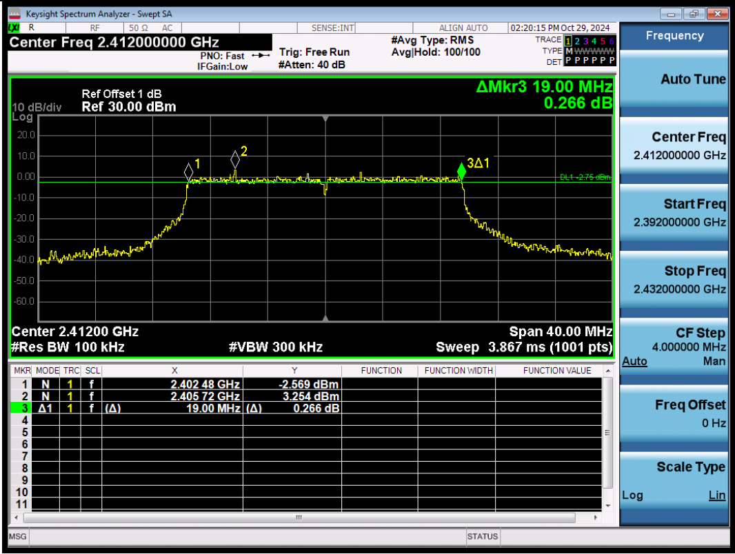
11AX20-2412-PASS
