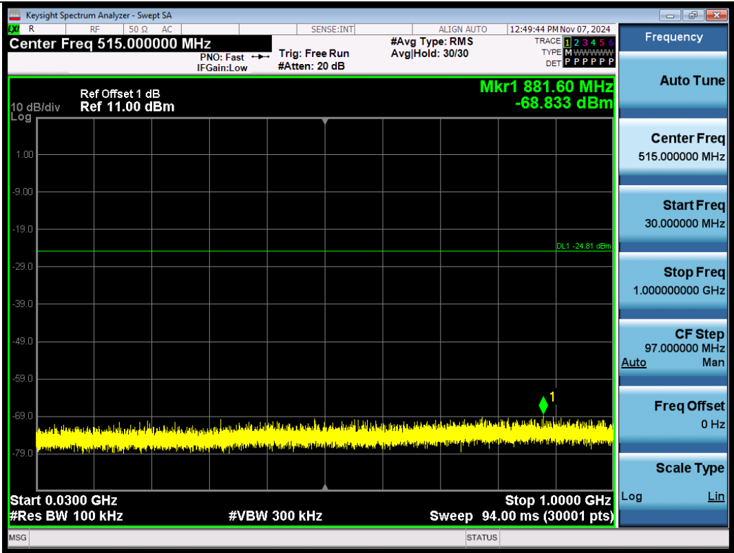
11B-2462-30~1000-PASS
