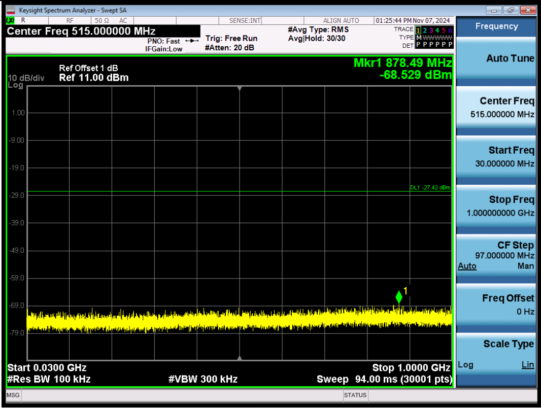
11G-2462-30~1000-PASS
