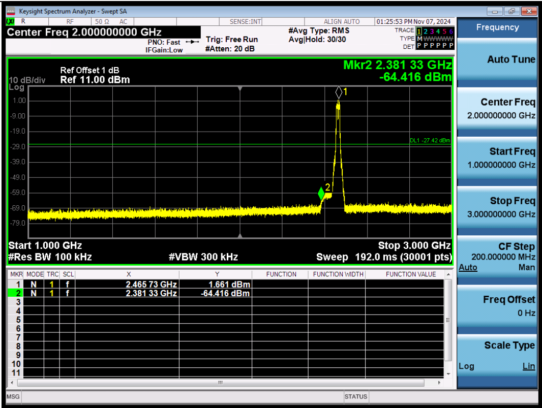
11G-2462-1000~3000-PASS
