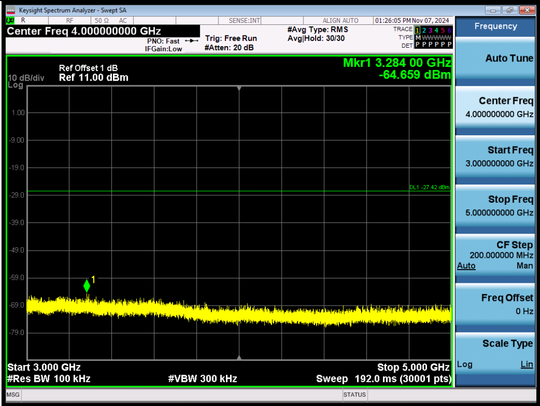
11G-2462-3000~5000-PASS
