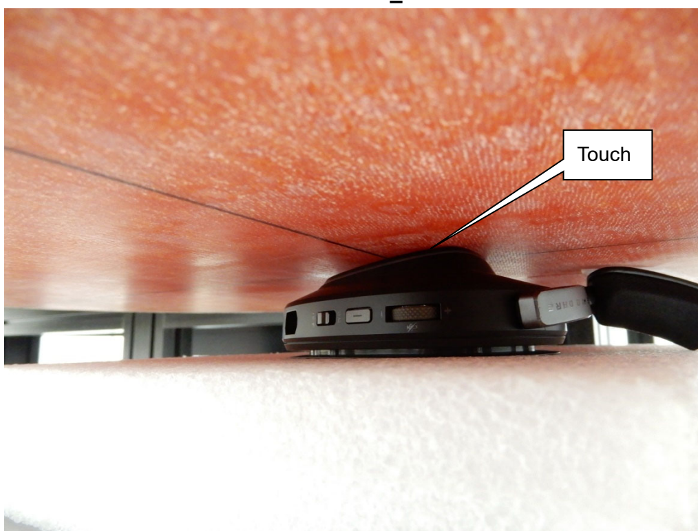
EUT Left-Ear_Back
