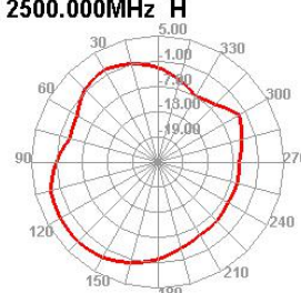
2500.000MHz H
