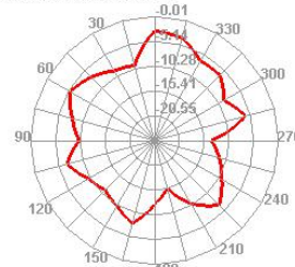
5100.000MHz E1
