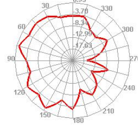
5500.000MHz E2
