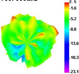
5900.000MHz
