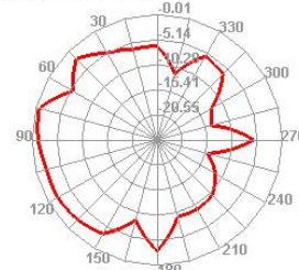
5100.000MHz E2
