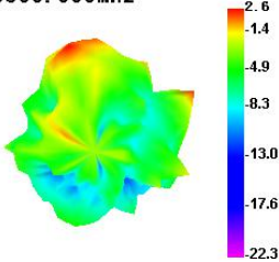
5500.000MHz
