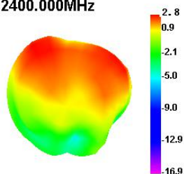
2400.000MHz
