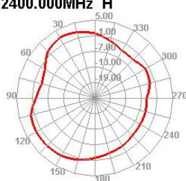
2400.000MHz H
