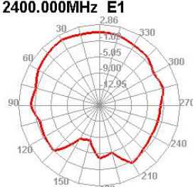
2400.000MHz E1
