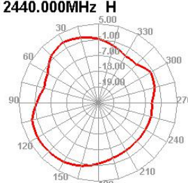
2440.000MHz H
