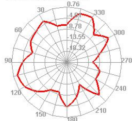
5900.000MHz E2
