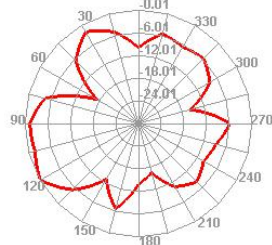
5100.000MHz H
