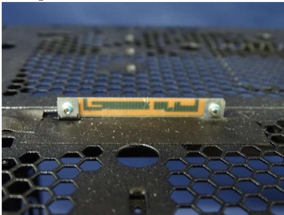
(44) EUT Photo_Antenna
