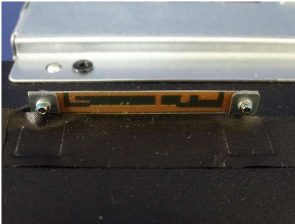
(42) EUT Photo_Antenna
