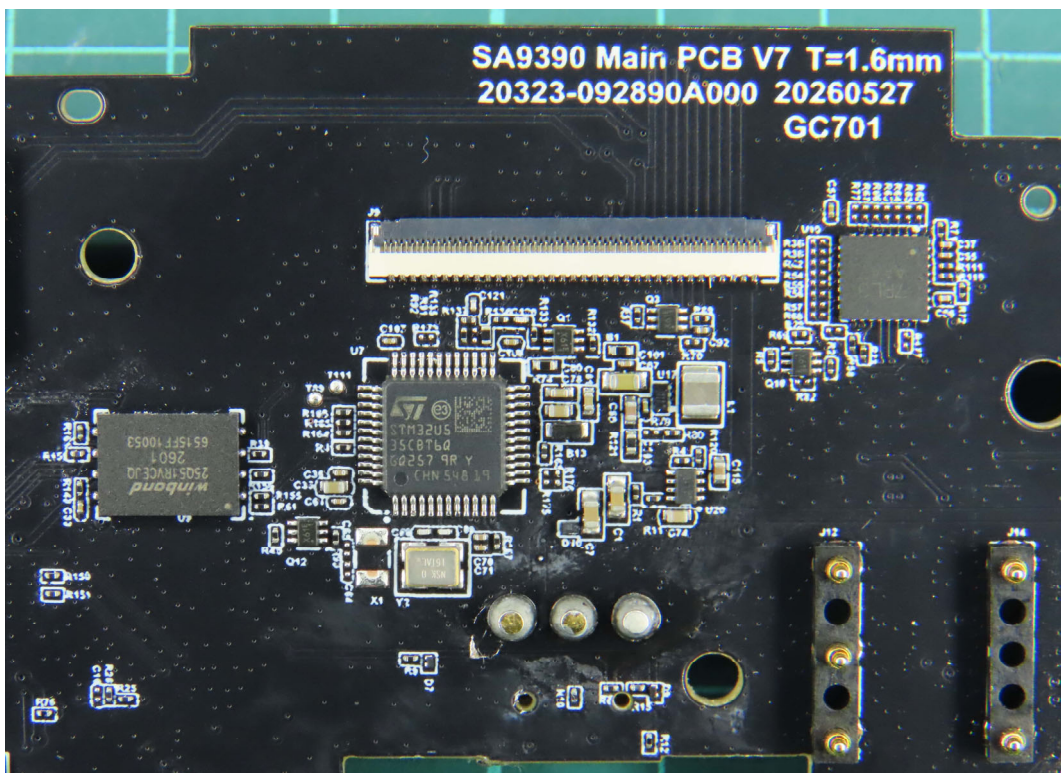
(59) EUT Photo
