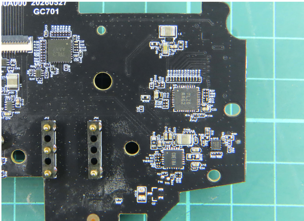
(61) EUT Photo
