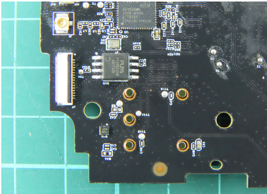
(53) EUT Photo
