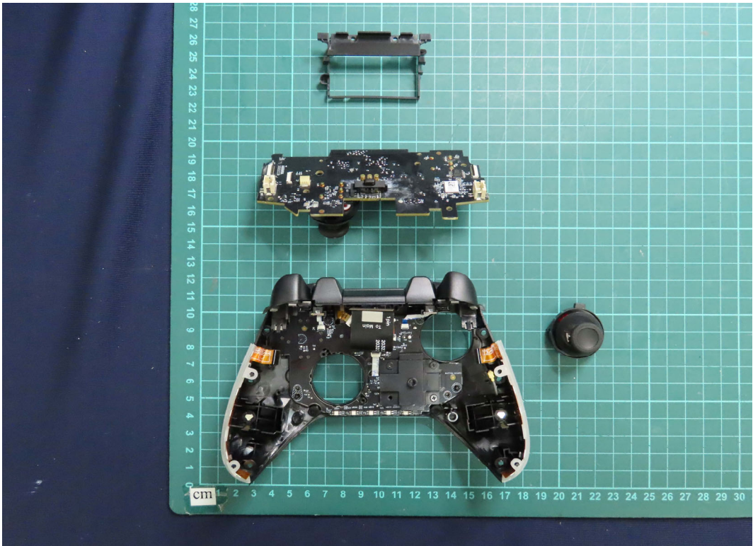
(49) EUT Photo
