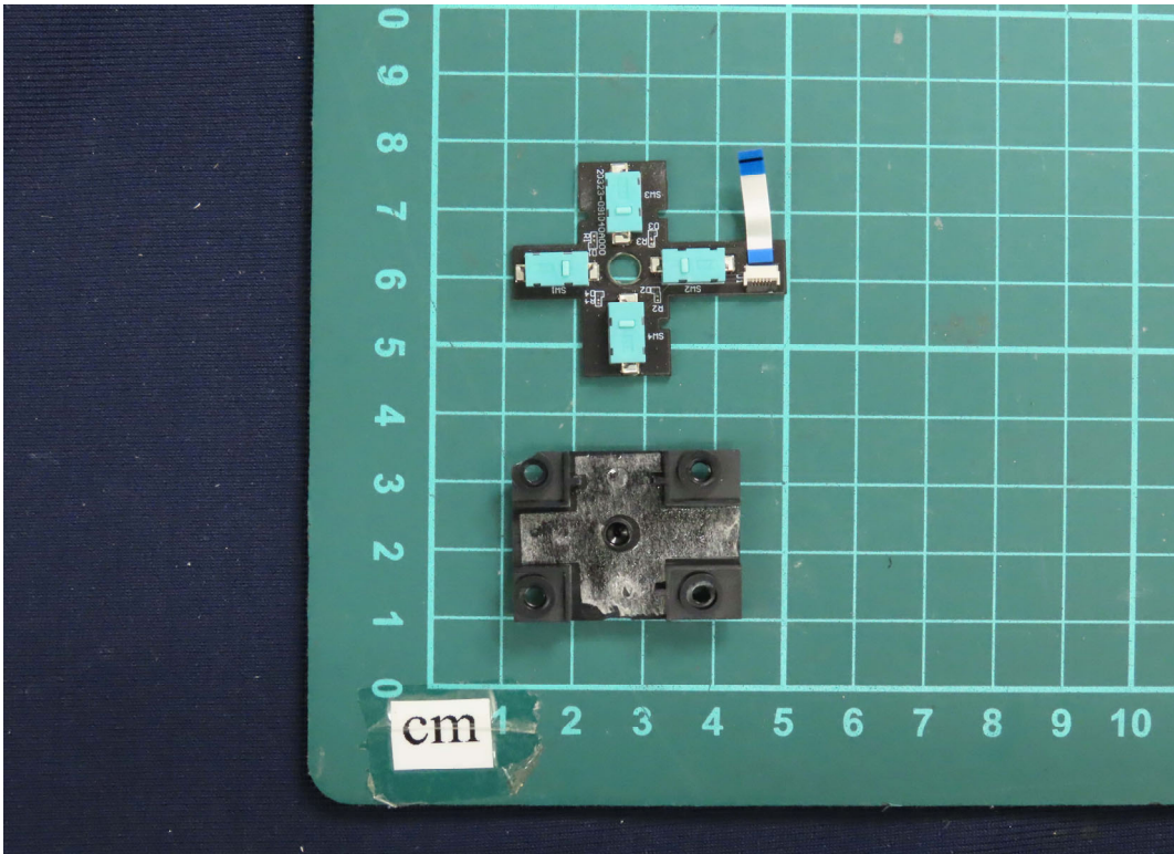
(67) EUT Photo
