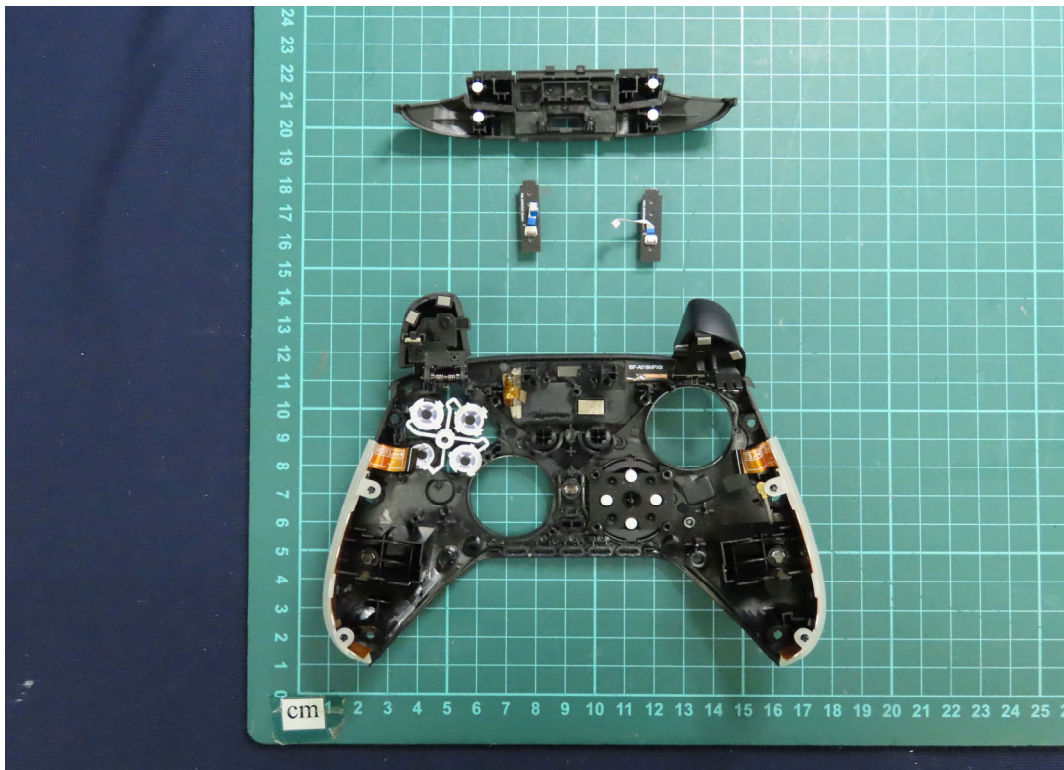
(71) EUT Photo
