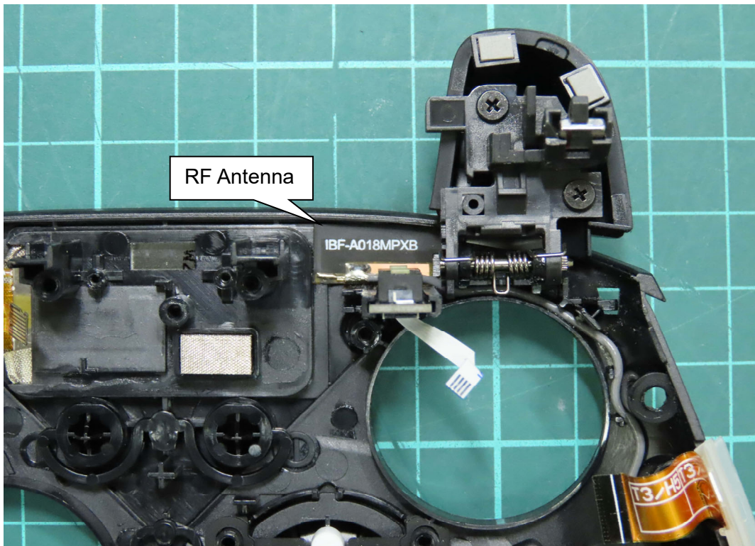
(75) EUT Photo
