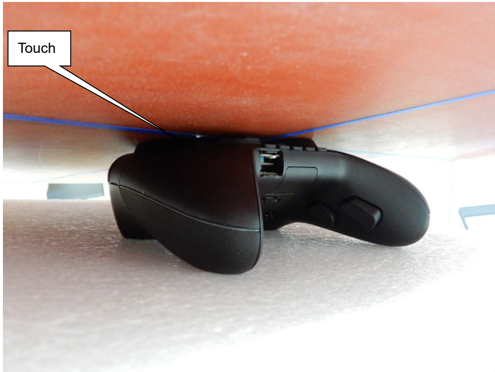
EUT Front
