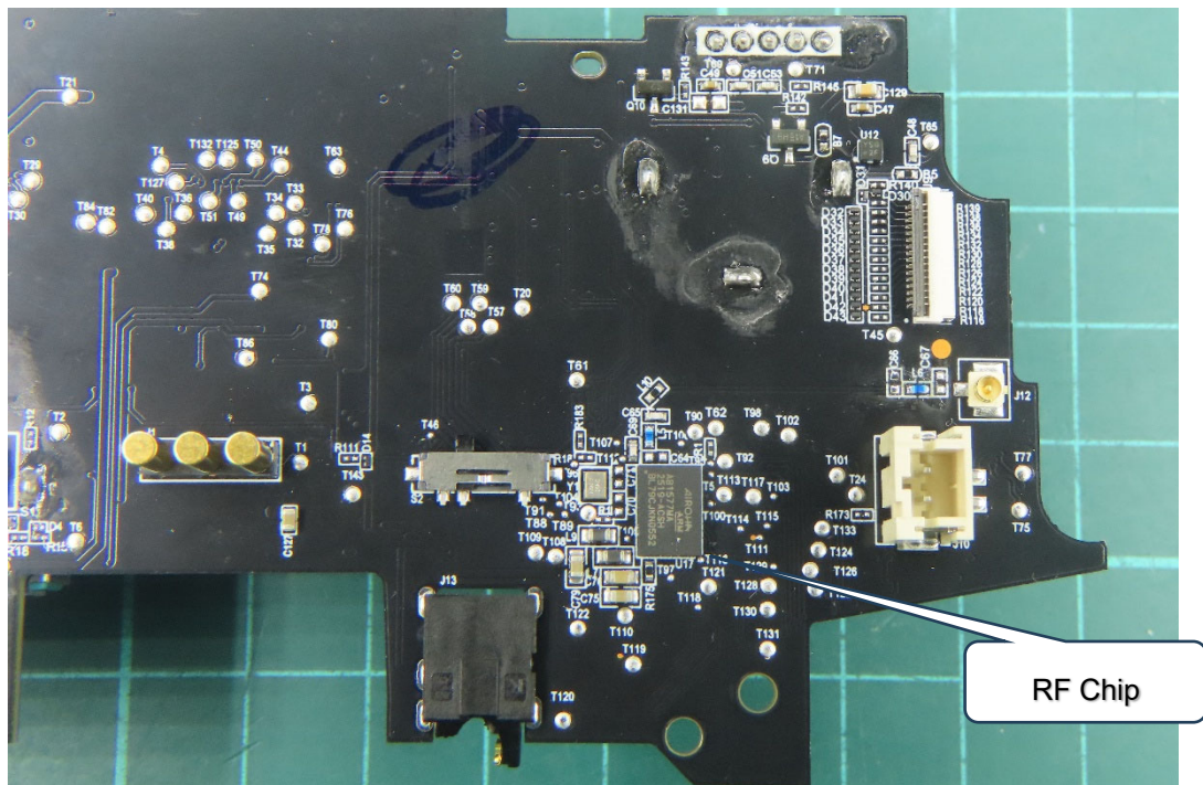
(9) EUT Photo
