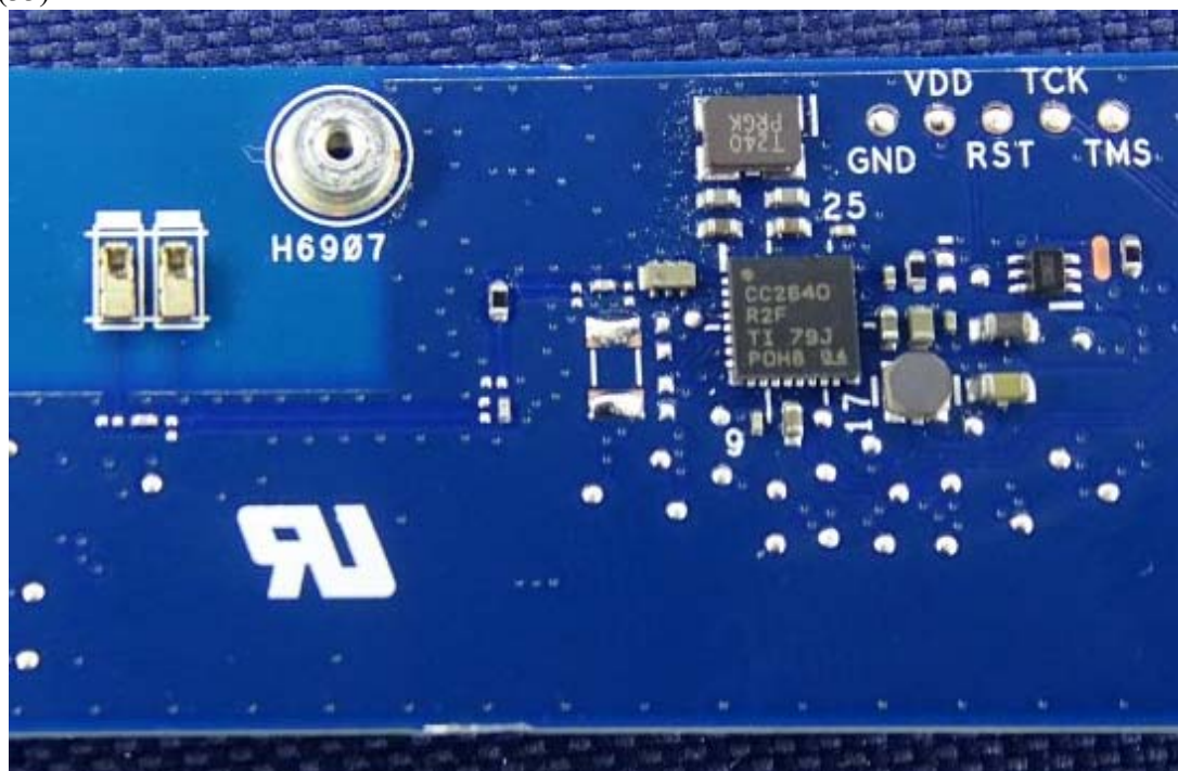
(33) EUT Photo
