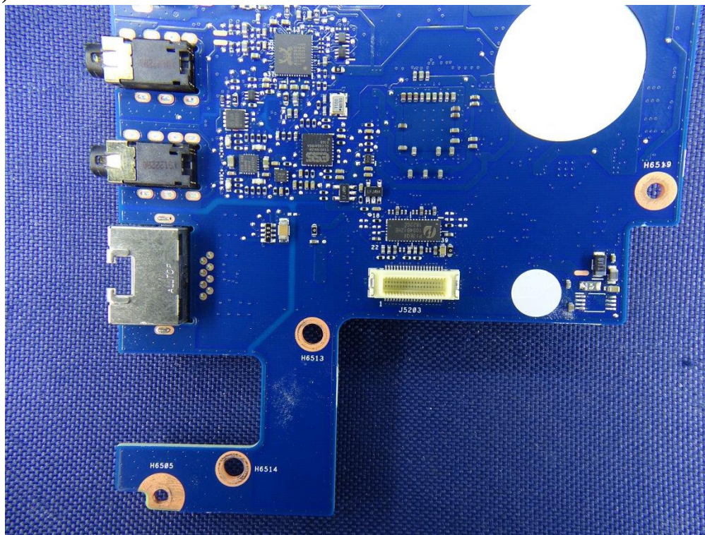
(54) EUT Photo
