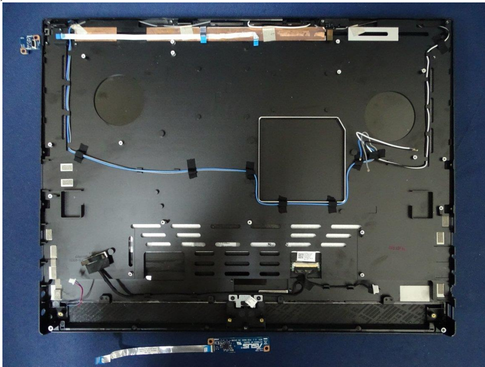
(64) EUT Photo
