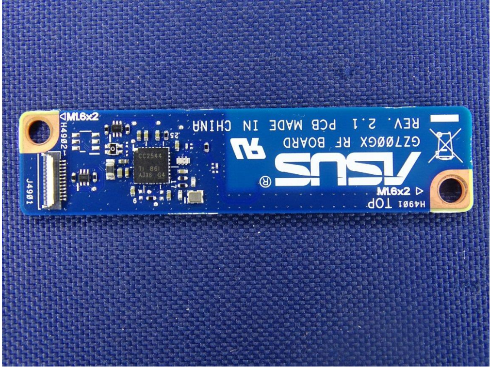
(66) EUT Photo
