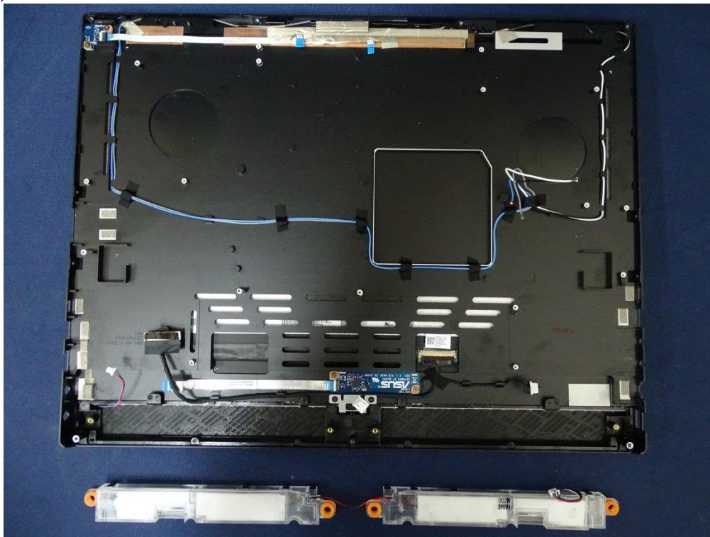
(63) EUT Photo
