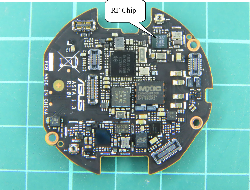
(21) EUT Photo
