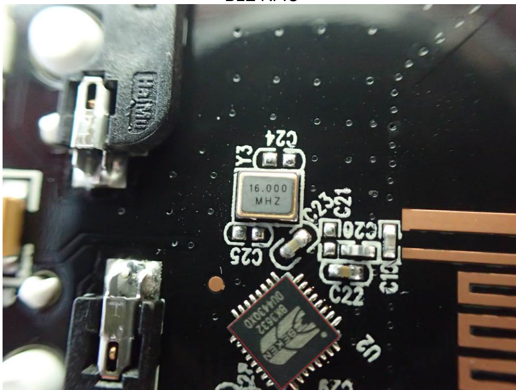
SRD2.4G RFIC
