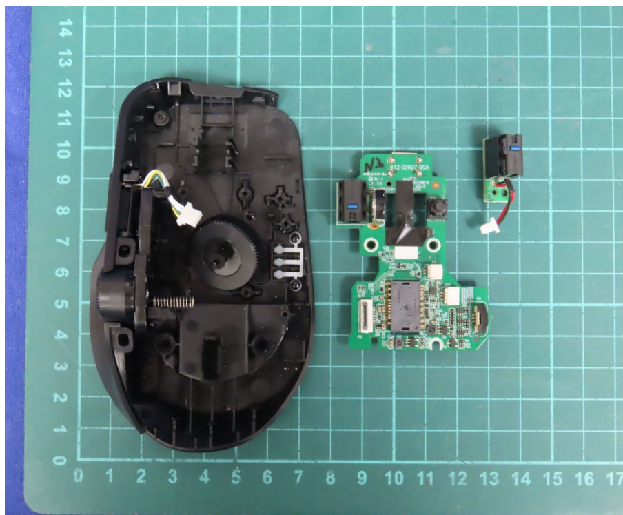
(13) EUT Photo
