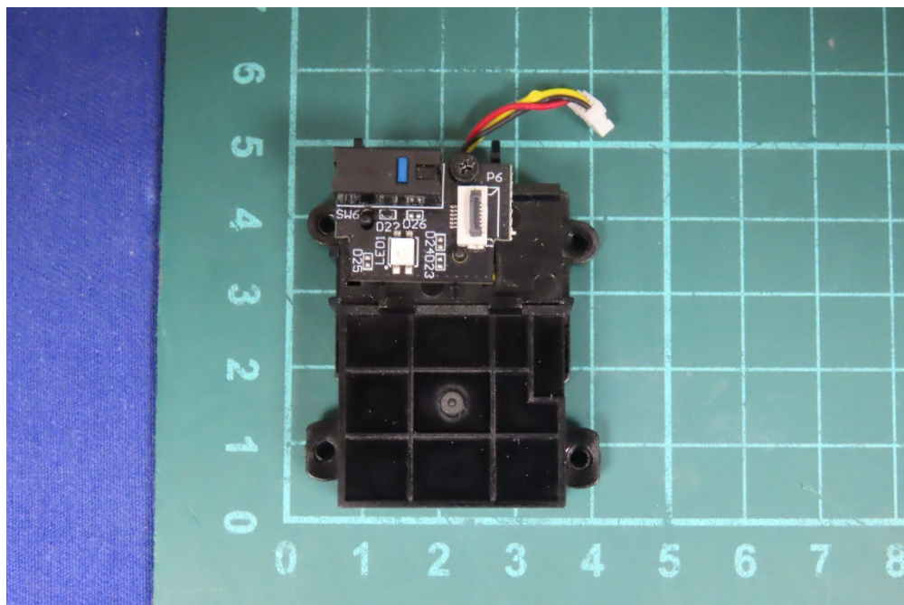
(6) EUT Photo
