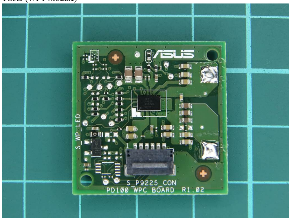
(10) EUT Photo (WPT Module)
