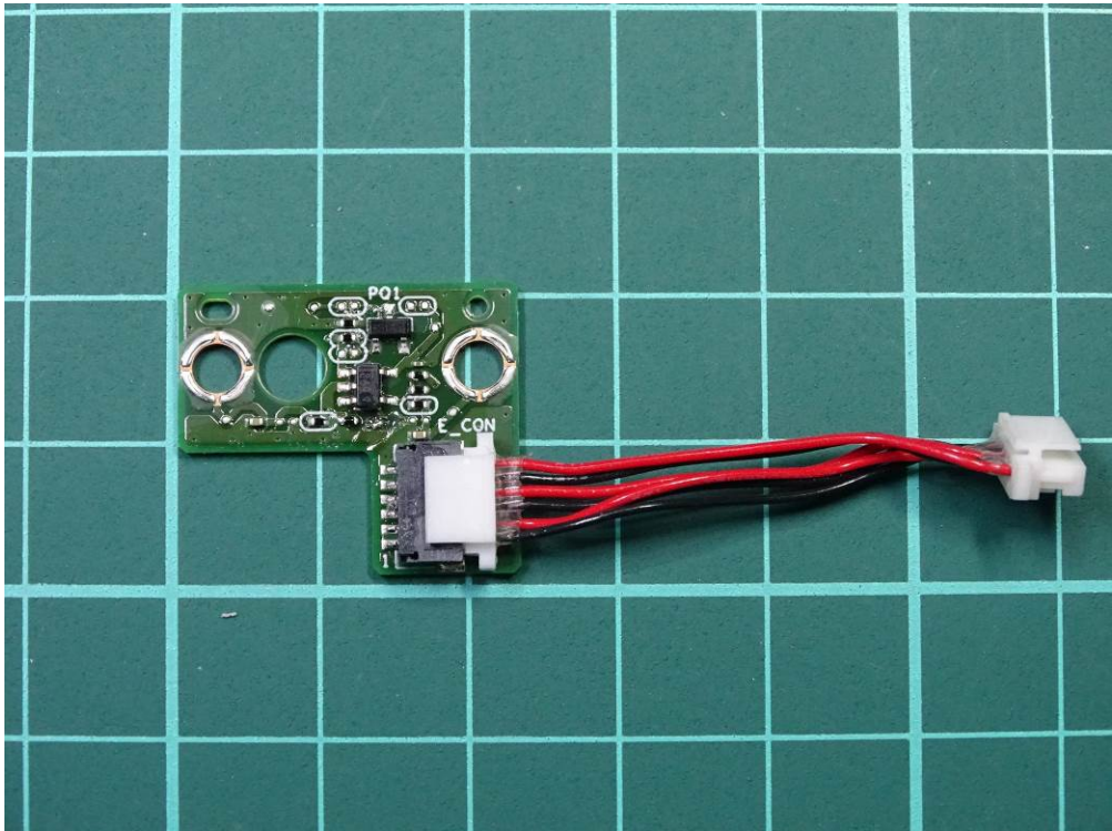
(36) EUT Photo
