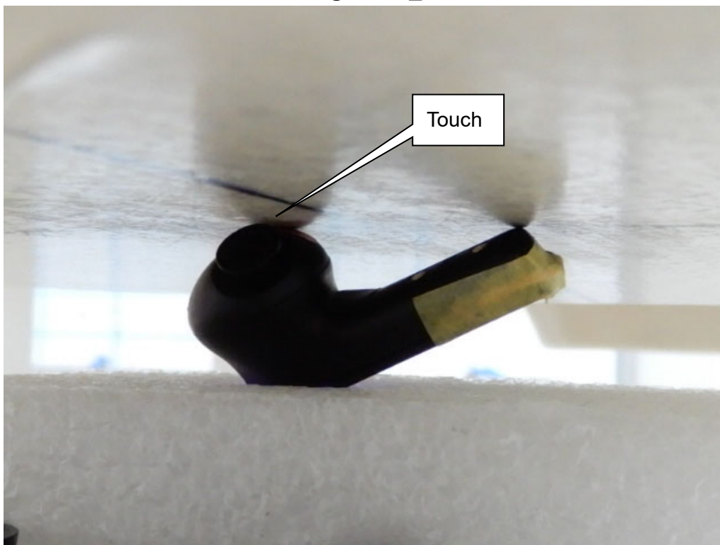
EUT Right-Ear_Back
