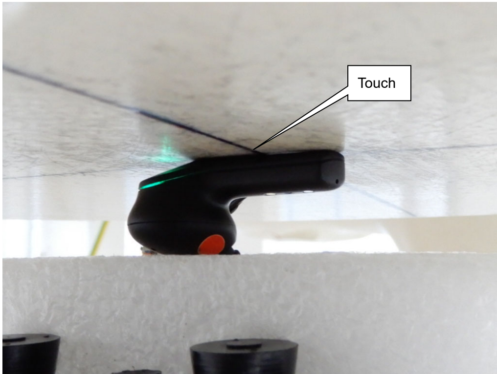
EUT Right-Ear_Front
