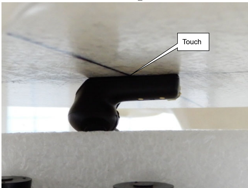
EUT Left-Ear_Front
