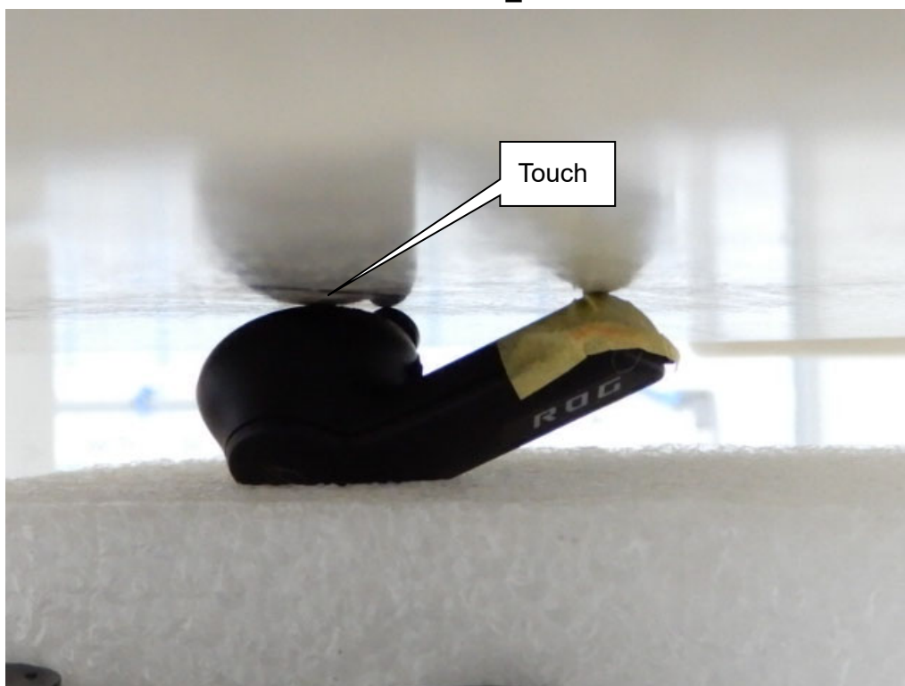
EUT Left-Ear_Back
