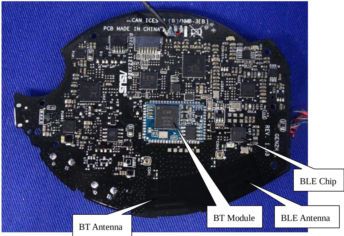
(21) EUT Photo
