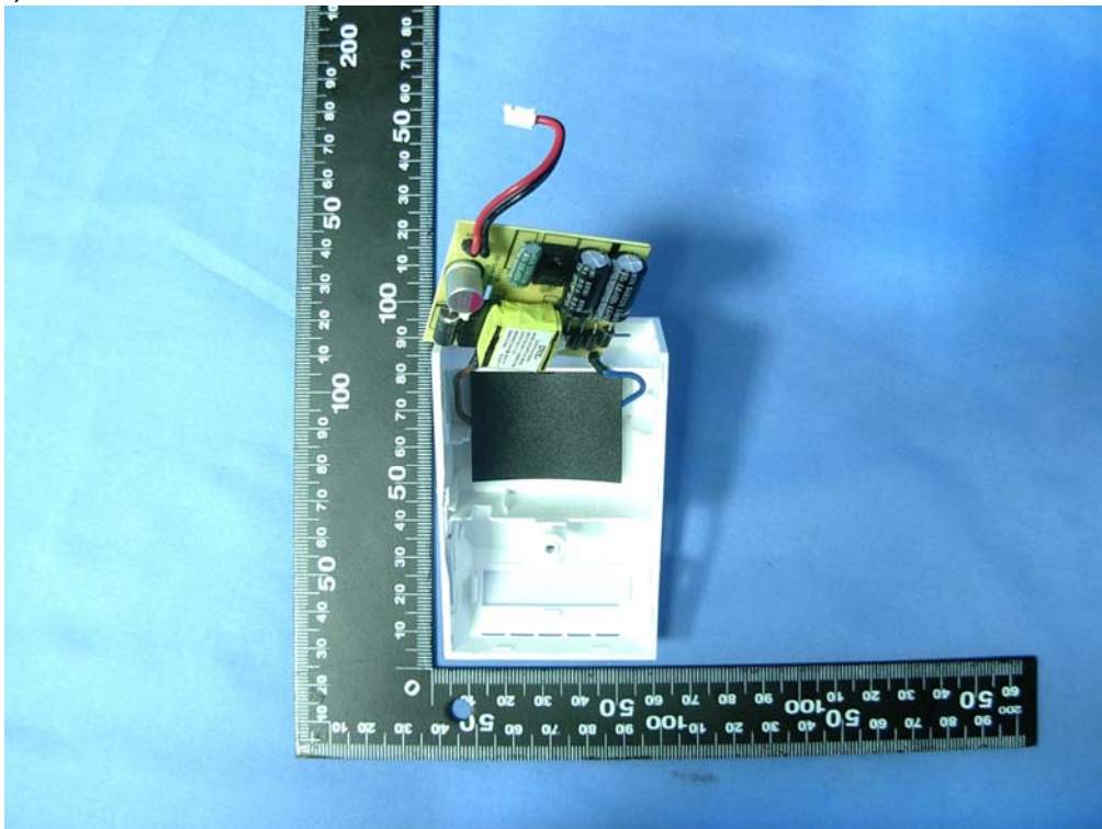
(20) EUT Photo
