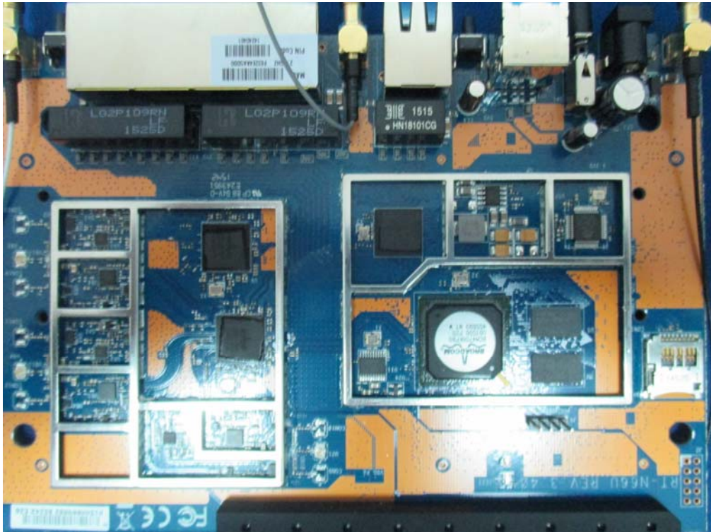
(17) EUT Photo
