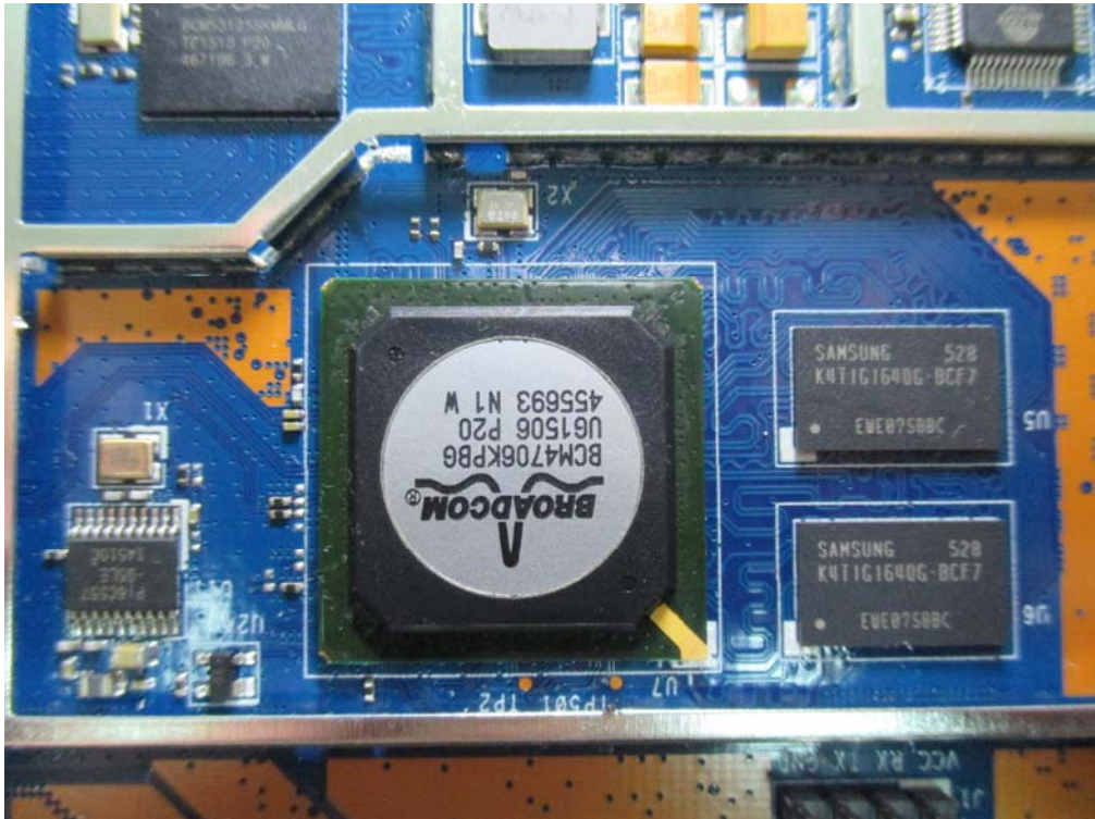
(31) EUT Photo
