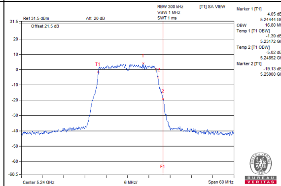
802.11a_Chain 1 / CH48
