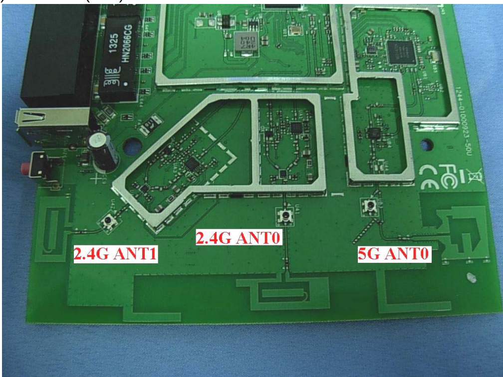
(15) EUT Photo (ANT)
