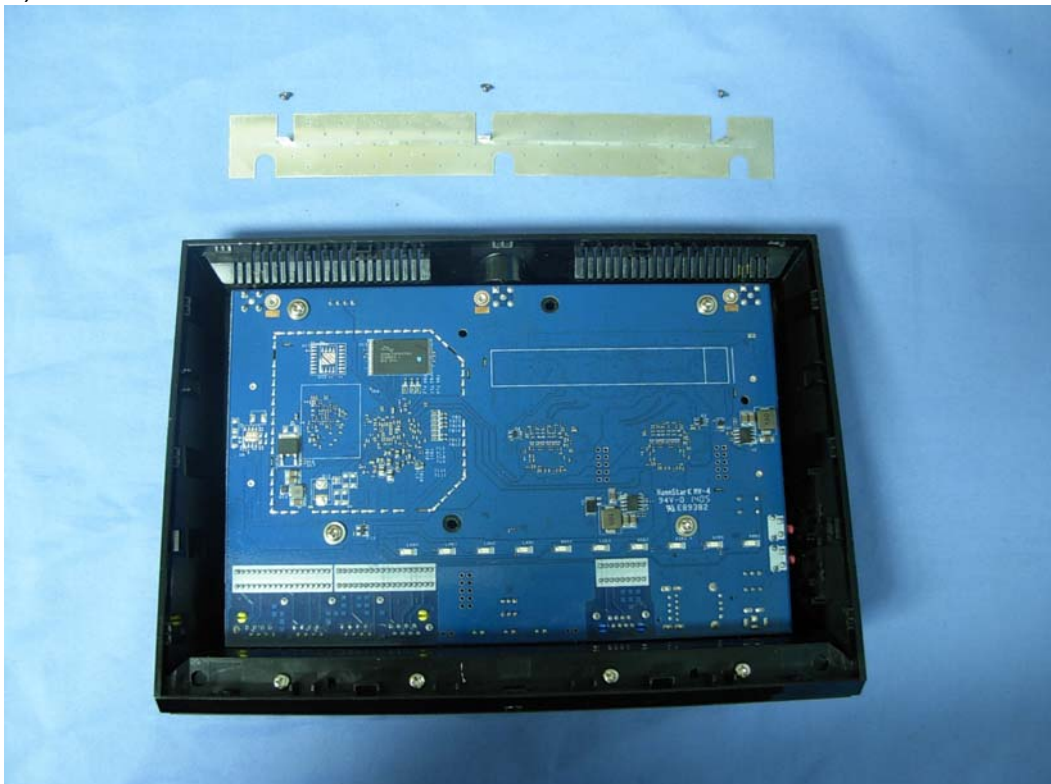
(36) EUT Photo
