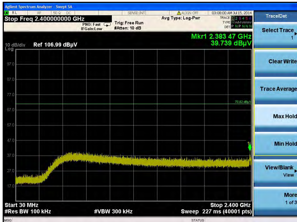
Plot on Configuration IEEE 802.11b / CH 11 / 30MHz~2400MHz (down 30dBc)
