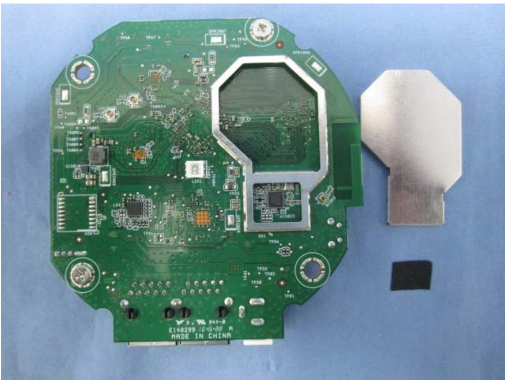
(4) EUT Photo
