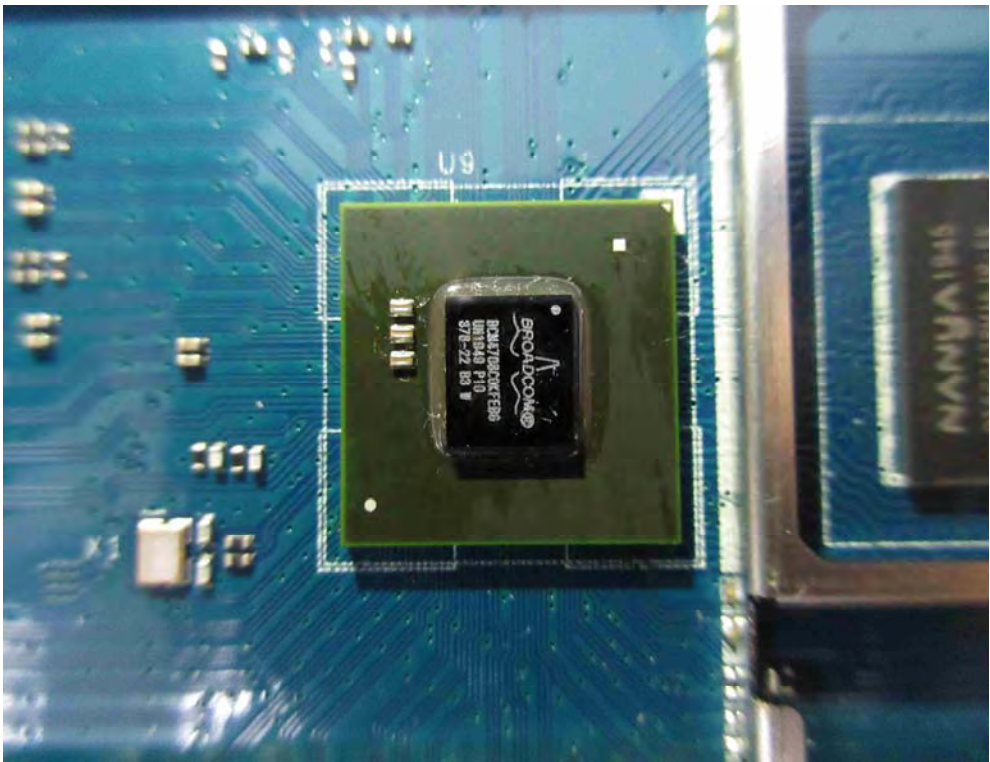
(24) EUT Photo
