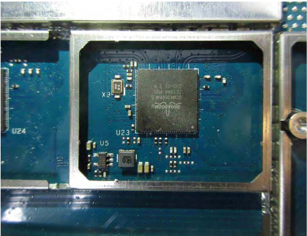
(30) EUT Photo
