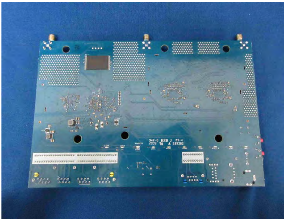
(6) EUT Photo
