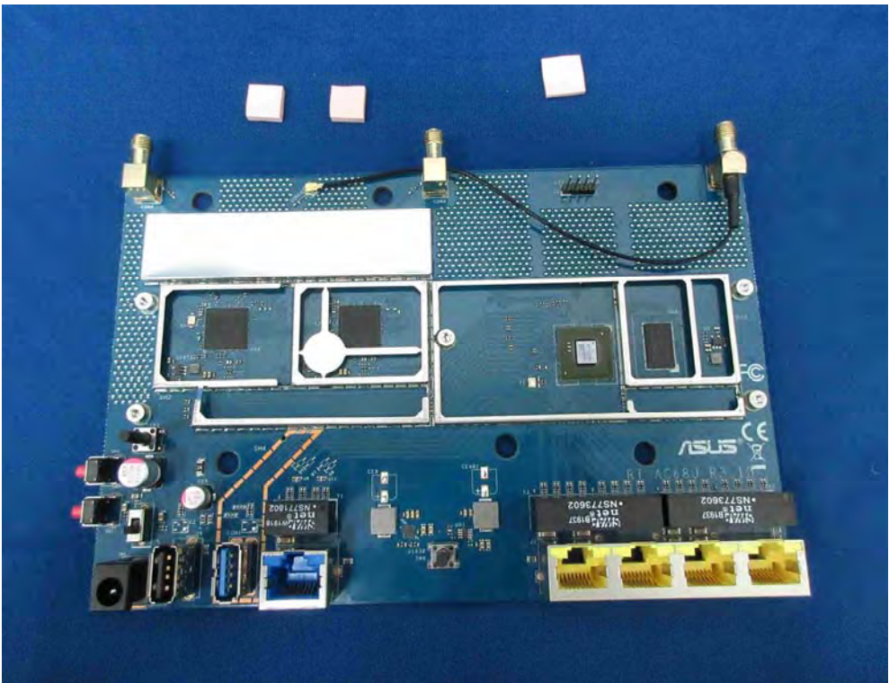
(20) EUT Photo
