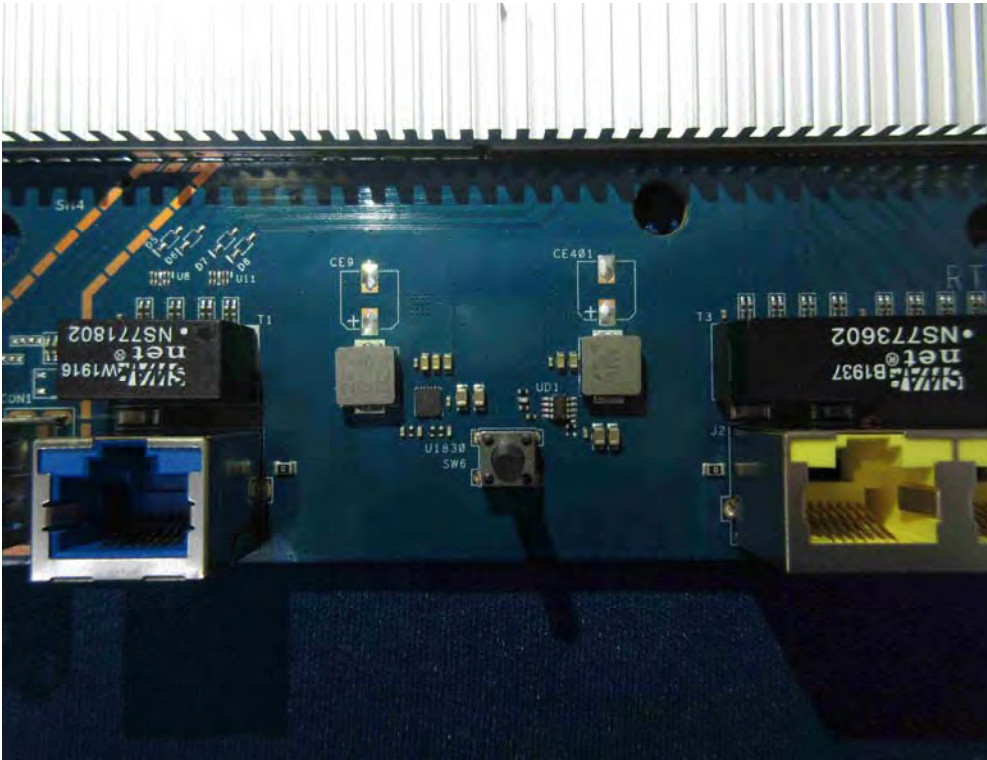
(16) EUT Photo
