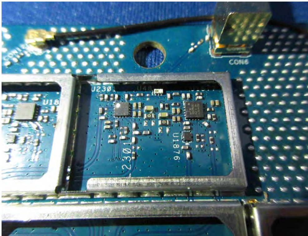
(36) EUT Photo
