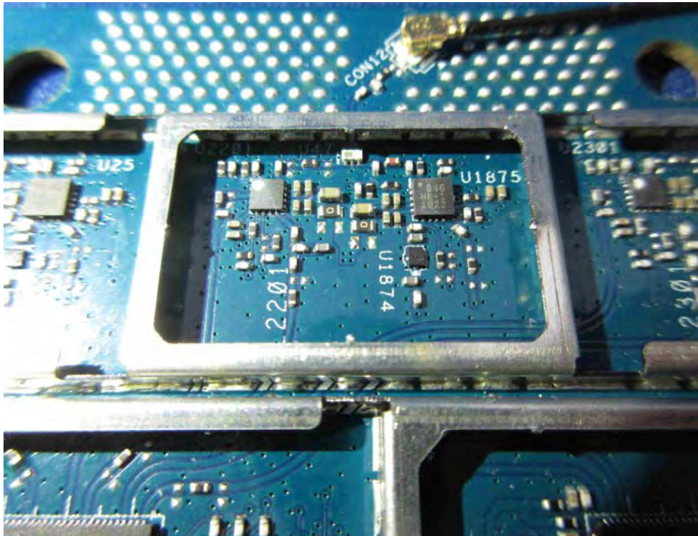
(36) EUT Photo
