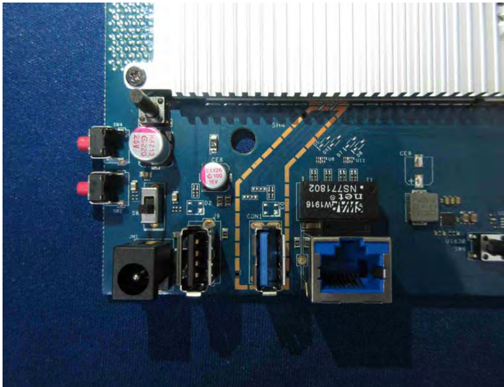
(14) EUT Photo
