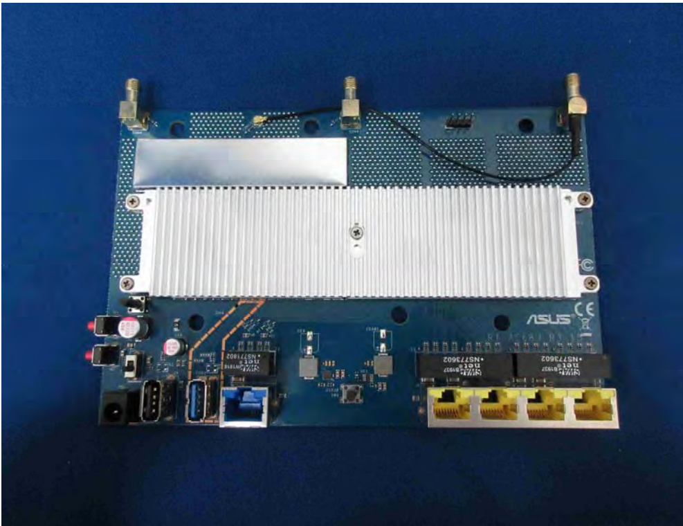
(4) EUT Photo
