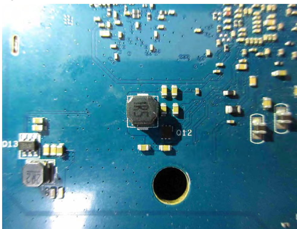
(8) EUT Photo
