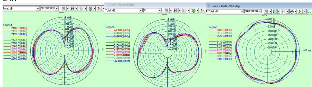
E1 (Phi=0)
