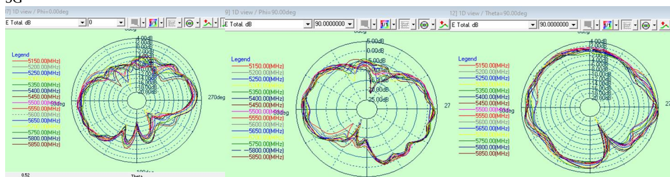
E1 (Phi=0)
