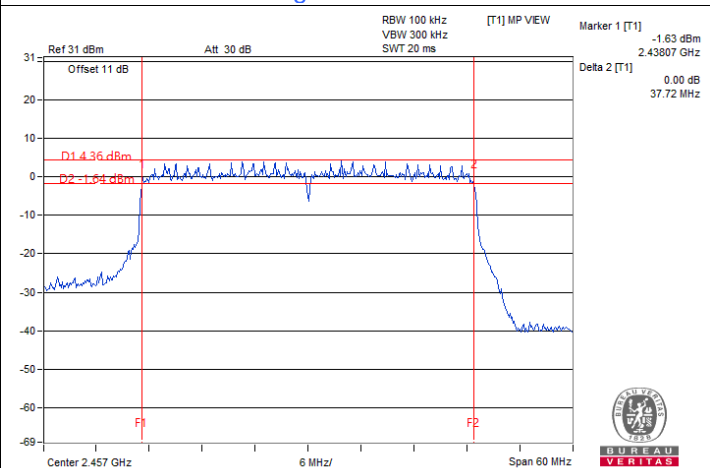
802.11ax (HE40) / Chain 0 : CH 10
