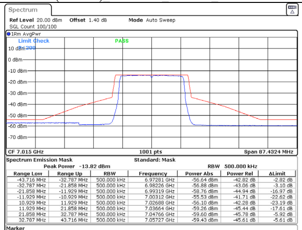
802.11ax (20MHz) 7015MHz Chain D NSS-2
