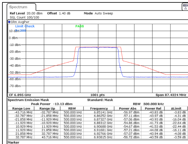
802.11ax (20MHz) 6895MHz Chain C NSS-2
