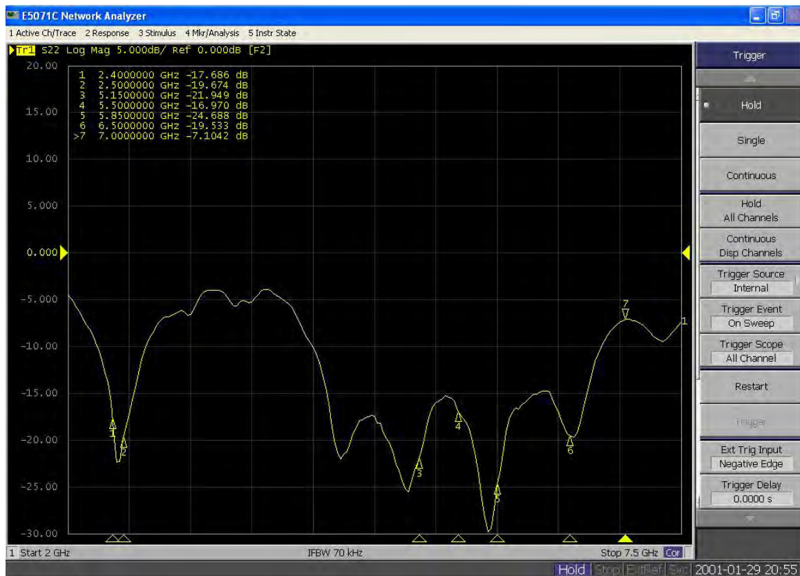
Figure 2、回波损耗截图
