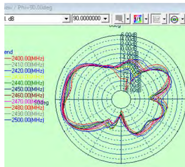
E2 (Phi=90)
