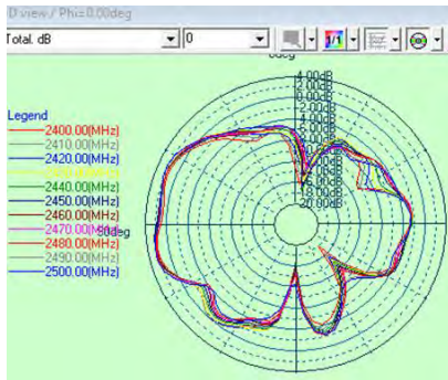
E1 (Phi=0)
