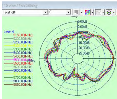
E1 (Phi=0)
