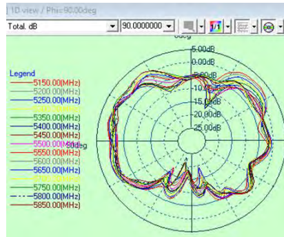
E2 (Phi=90)
