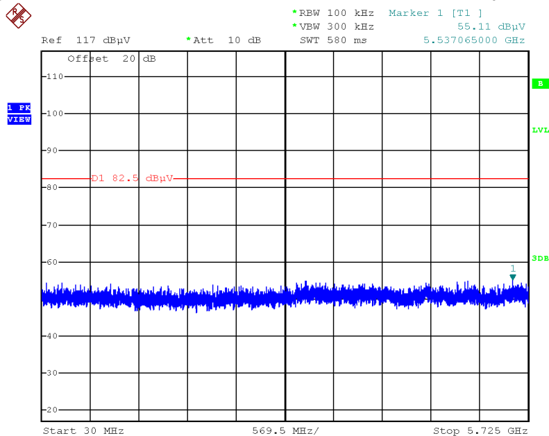
Plot on Configuration IEEE 802.11ac MCS0/Nss1 VHT20 / CH 165 / 30MHz~5725MHz (down 30dBc)
