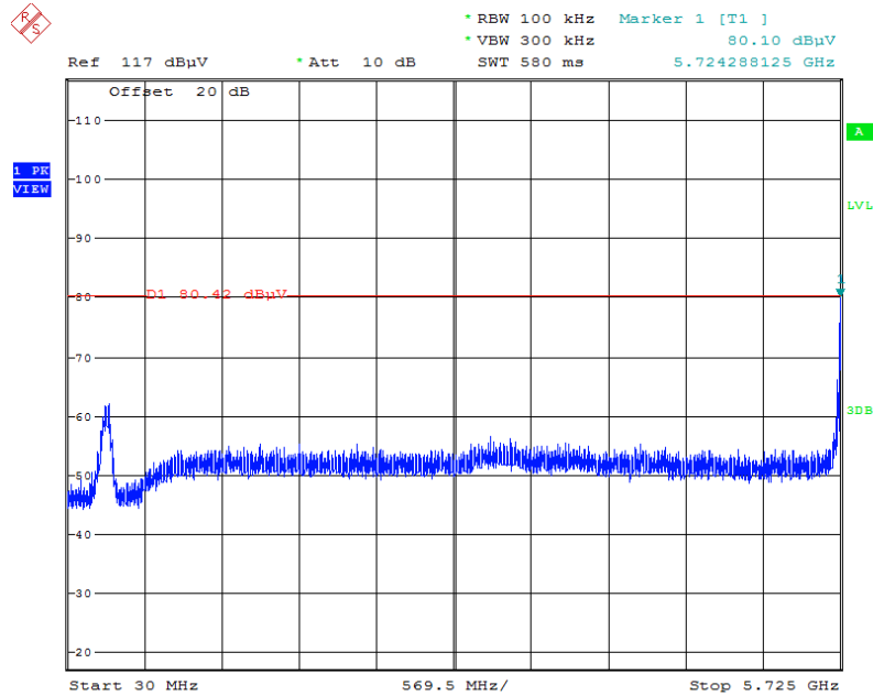
Plot on Configuration IEEE 802.11ac MCS0/Nss1 VHT40 / CH 151 / 30MHz~5725MHz (down 30dBc)
