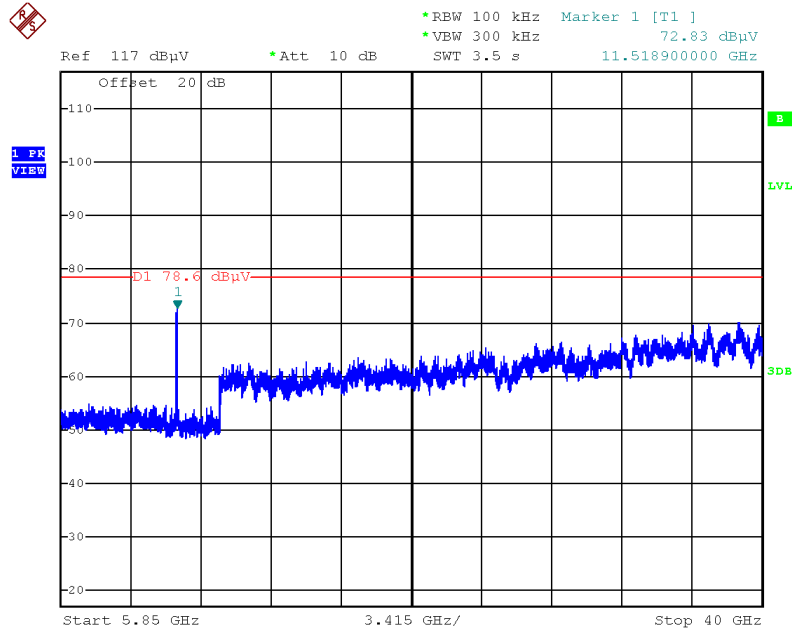
Plot on Configuration IEEE 802.11ac MCS0/Nss2 VHT40 / CH 151 / 5850MHz~40000MHz (down 30dBc)
