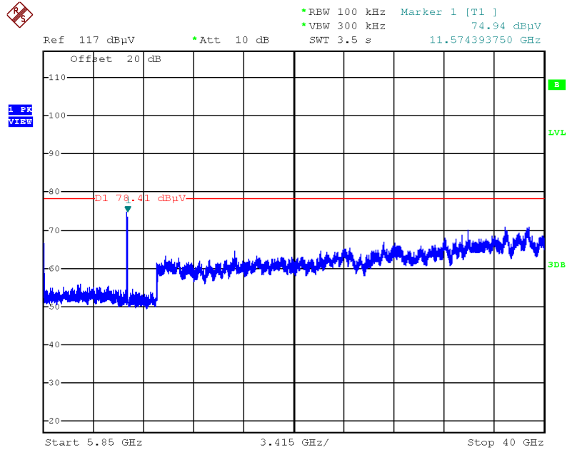
Plot on Configuration IEEE 802.11ac MCS0/Nss1 VHT40 / CH 159 / 5850MHz~40000MHz (down 30dBc)
