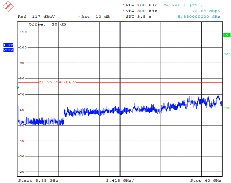
Plot on Configuration IEEE 802.11ac MCS0/Nss1 VHT80 / CH 155 / 5850MHz~40000MHz (down 30dBc)
