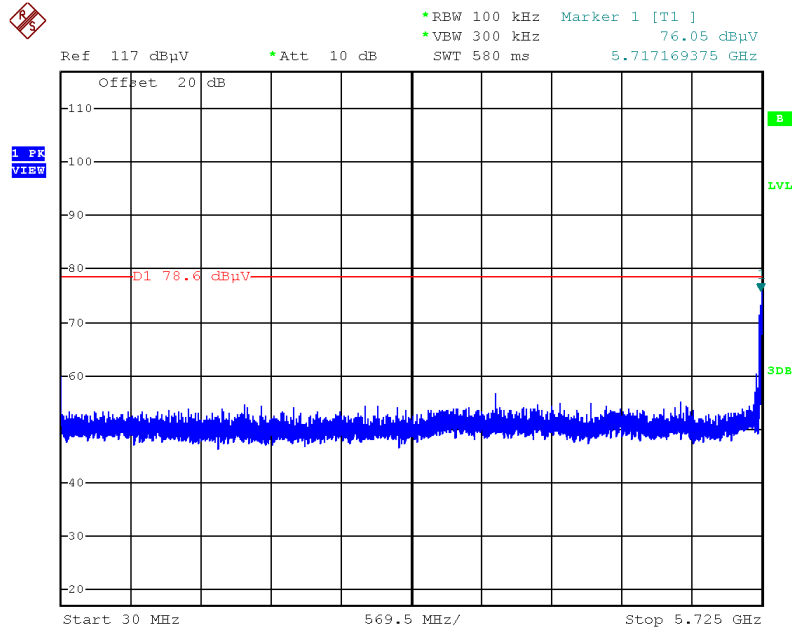
Plot on Configuration IEEE 802.11ac MCS0/Nss2 VHT40 / CH 151 / 30MHz~5725MHz (down 30dBc)
