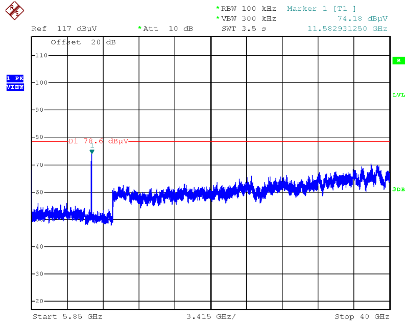
Plot on Configuration IEEE 802.11ac MCS0/Nss2 VHT40 / CH 159 / 5850MHz~40000MHz (down 30dBc)
