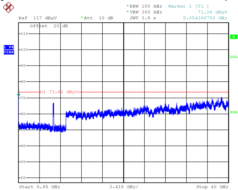
Plot on Configuration IEEE 802.11ac MCS0/Nss2 VHT80 / CH 155 / 5850MHz~40000MHz (down 30dBc)
