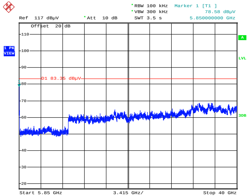
Plot on Configuration IEEE 802.11ac MCS0/Nss4 VHT 80 / CH 155 / 5850MHz~40000MHz (down 30dBc)
