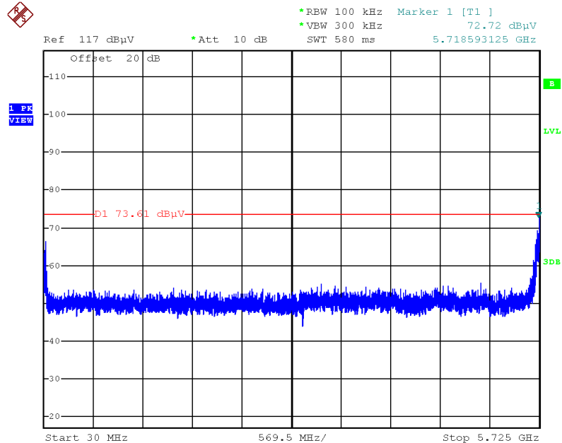
Plot on Configuration IEEE 802.11ac MCS0/Nss2 VHT80 / CH 155 / 30MHz~5725MHz (down 30dBc)
