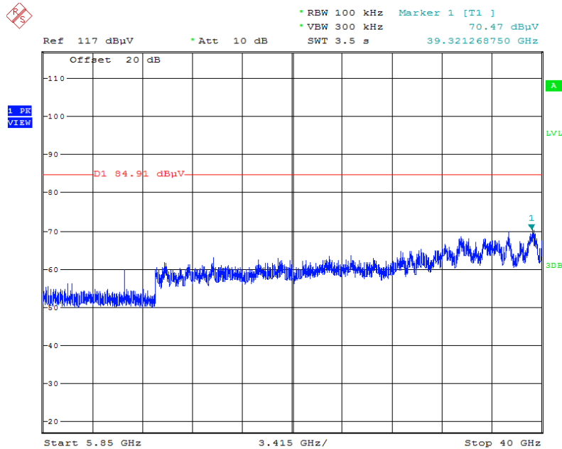
Plot on Configuration IEEE 802.11ac MCS0/Nss1 VHT20 / CH 149 / 5850MHz~40000MHz (down 30dBc)
