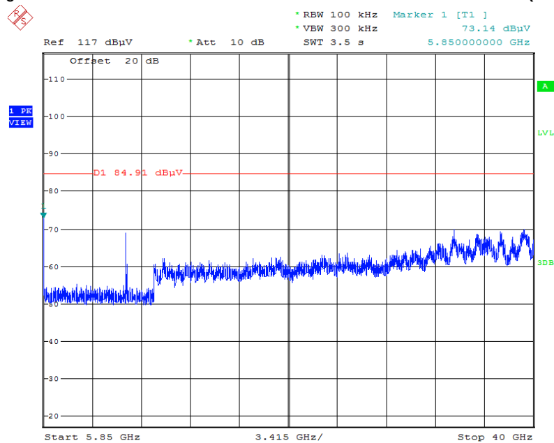
Plot on Configuration IEEE 802.11ac MCS0/Nss1 VHT20 / CH 165 / 5850MHz~40000MHz (down 30dBc)
