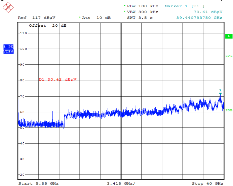
Plot on Configuration IEEE 802.11ac MCS0/Nss1 VHT40 / CH 159 / 5850MHz~40000MHz (down 30dBc)
