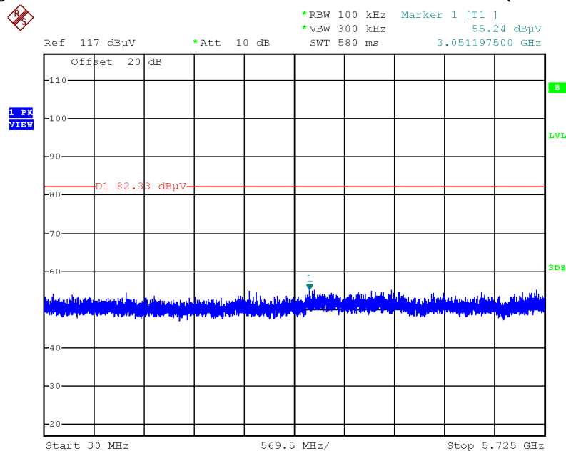
Plot on Configuration IEEE 802.11ac MCS0/Nss2 VHT20 / CH 165 / 30MHz~5725MHz (down 30dBc)
