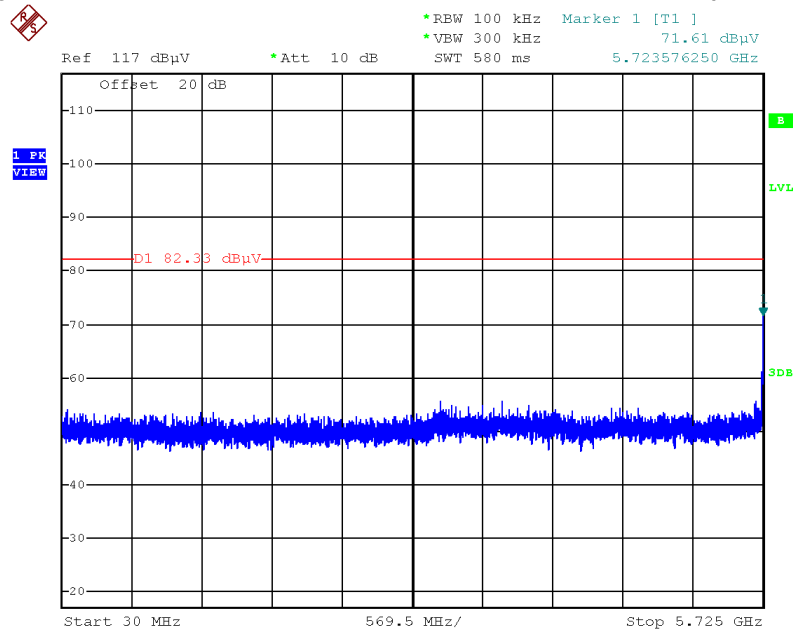
Plot on Configuration IEEE 802.11ac MCS0/Nss2 VHT20 / CH 149 / 30MHz~5725MHz (down 30dBc)
