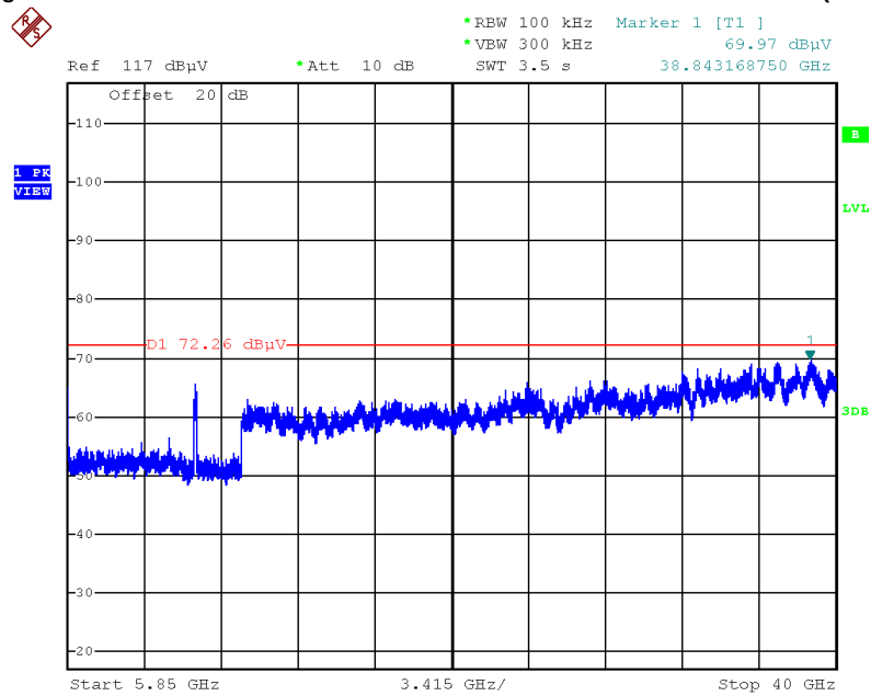
Plot on Configuration IEEE 802.11ac MCS0/Nss1 VHT80 / CH 155 / 5850MHz~40000MHz (down 30dBc)
