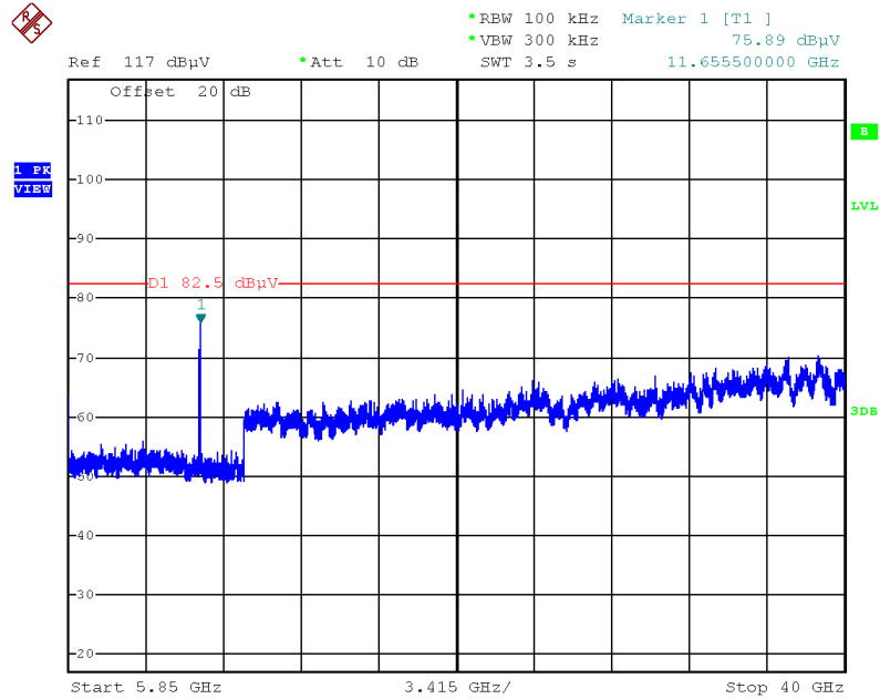
Plot on Configuration IEEE 802.11ac MCS0/Nss1 VHT20 / CH 165 / 5850MHz~40000MHz (down 30dBc)
