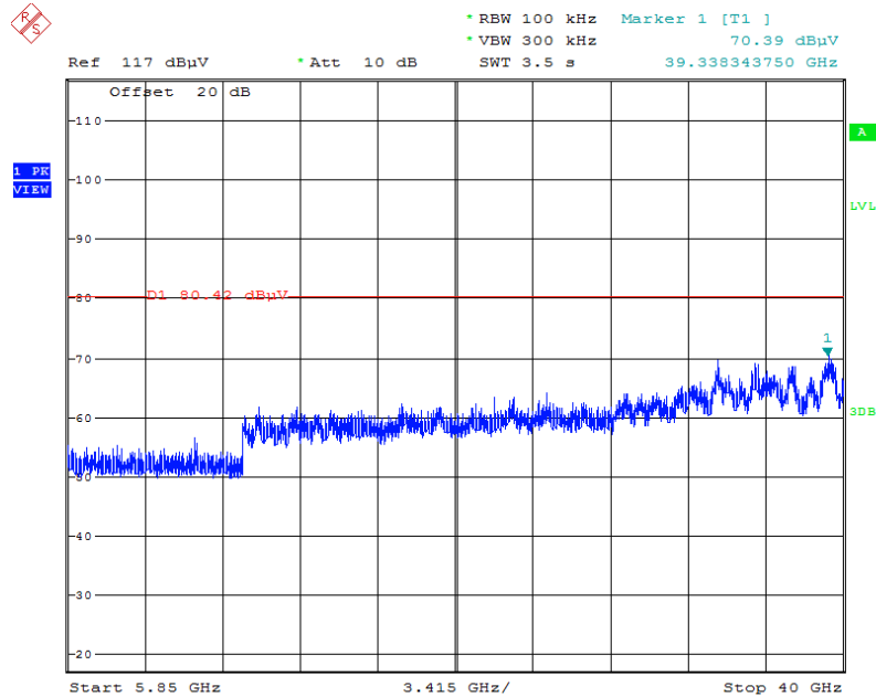
Plot on Configuration IEEE 802.11ac MCS0/Nss1 VHT40 / CH 151 / 5850MHz~40000MHz (down 30dBc)
