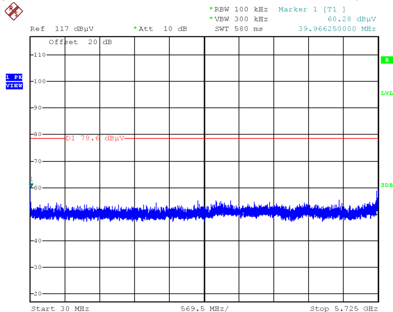
Plot on Configuration IEEE 802.11ac MCS0/Nss2 VHT40 / CH 159 / 30MHz~5725MHz (down 30dBc)
