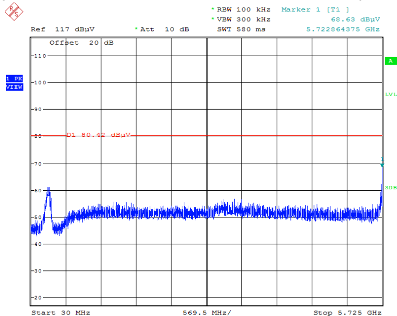
Plot on Configuration IEEE 802.11ac MCS0/Nss1 VHT40 / CH 159 / 30MHz~5725MHz (down 30dBc)
