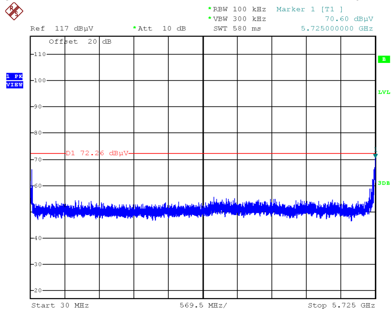
Plot on Configuration IEEE 802.11ac MCS0/Nss1 VHT80 / CH 155 / 30MHz~5725MHz (down 30dBc)
