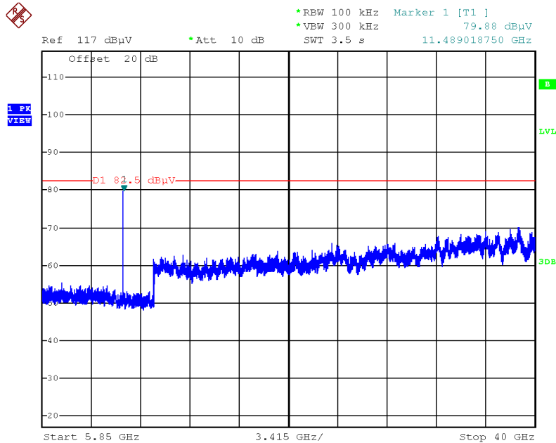
Plot on Configuration IEEE 802.11ac MCS0/Nss1 VHT20 / CH 149 / 5850MHz~40000MHz (down 30dBc)
