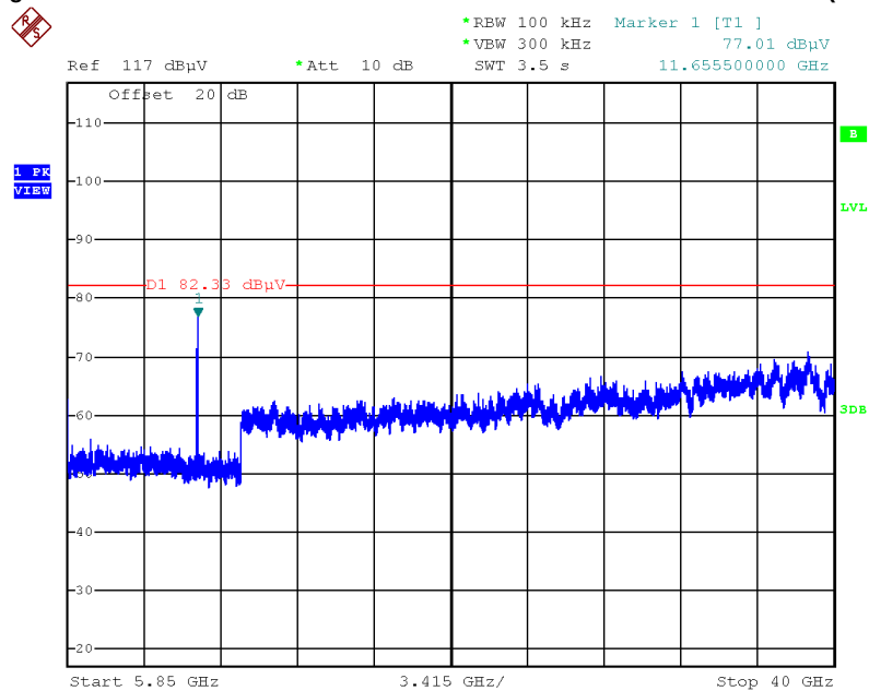
Plot on Configuration IEEE 802.11ac MCS0/Nss2 VHT20 / CH 165 / 5850MHz~40000MHz (down 30dBc)
