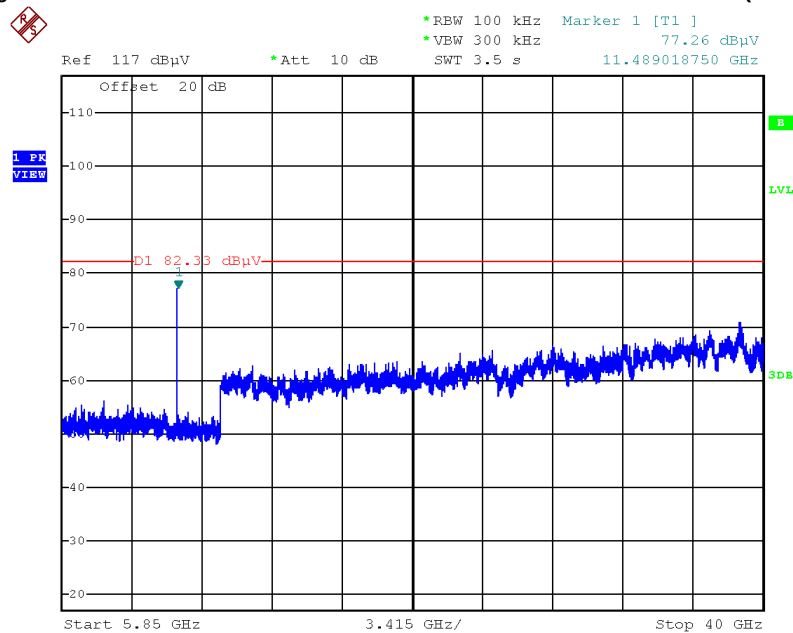
Plot on Configuration IEEE 802.11ac MCS0/Nss2 VHT20 / CH 149 / 5850MHz~40000MHz (down 30dBc)
