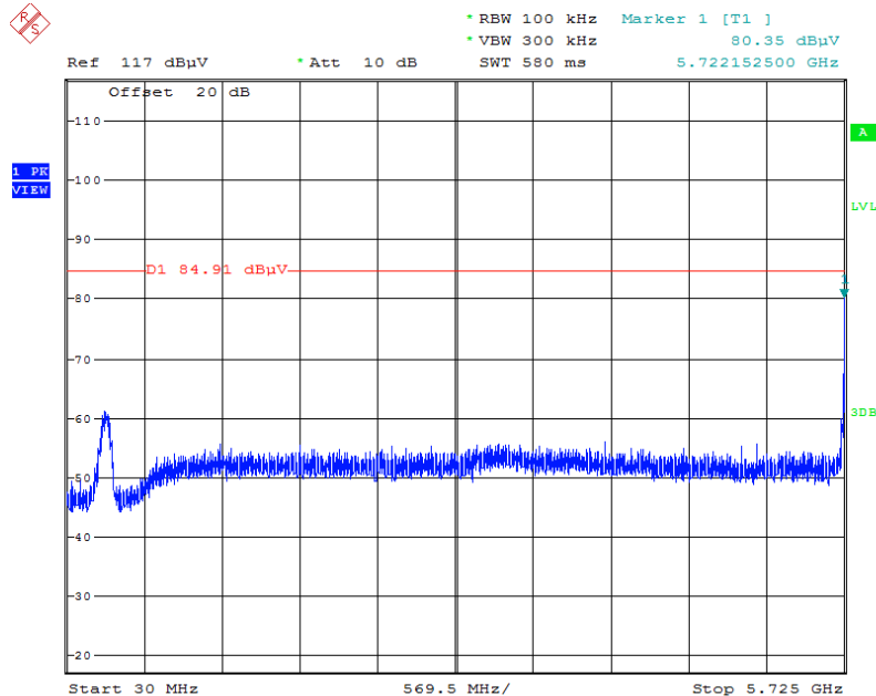
Plot on Configuration IEEE 802.11ac MCS0/Nss1 VHT20 / CH 149 / 30MHz~5725MHz (down 30dBc)
