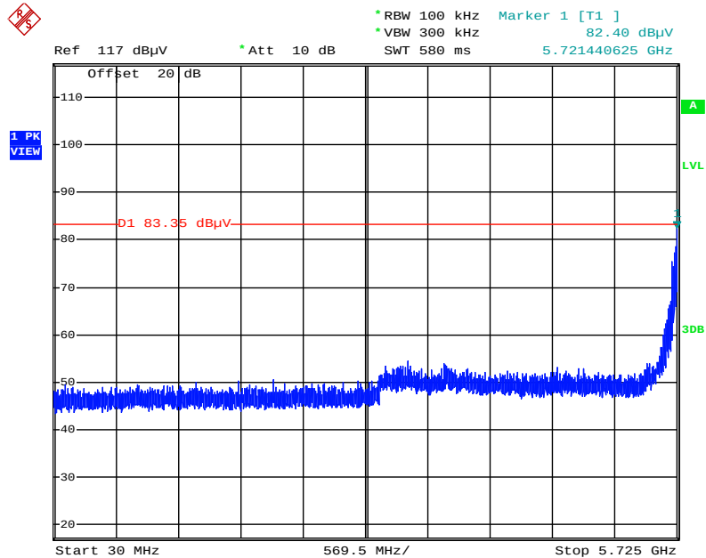
Plot on Configuration IEEE 802.11ac MCS0/Nss4 VHT 80 / CH 155 / 30MHz~5725MHz (down 30dBc)
