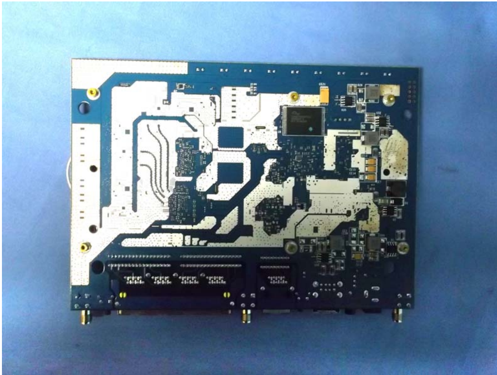
(31) EUT Photo
