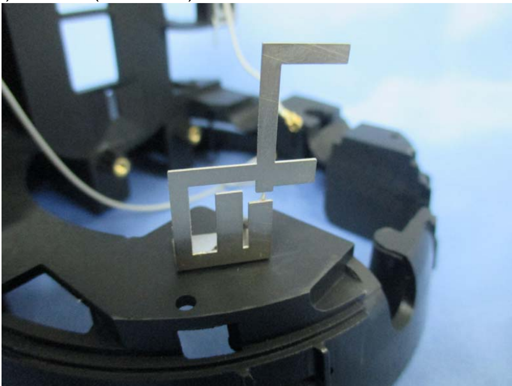
(48) EUT Photo (Antenna AUX)
