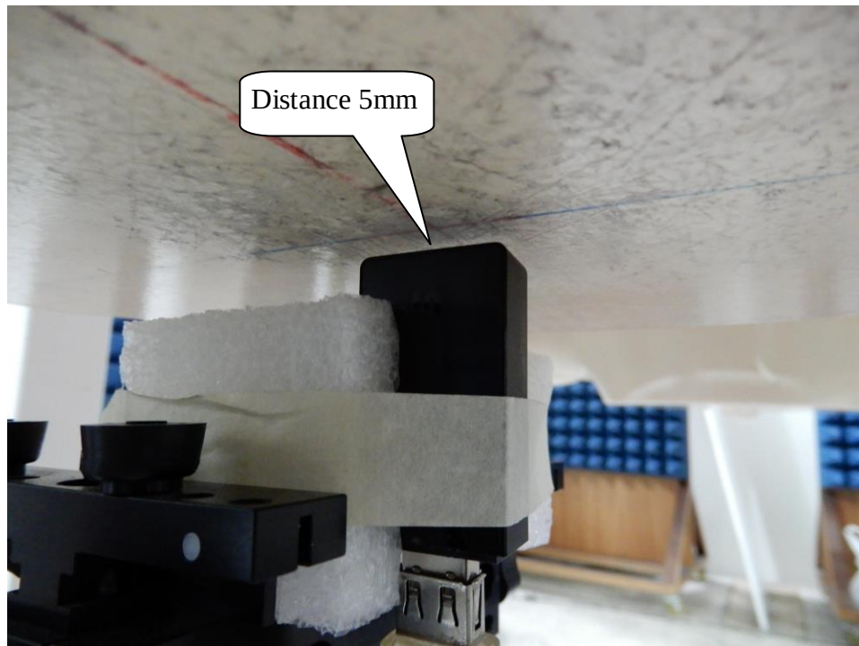
EUT Tip
