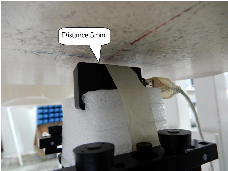
EUT Right-Side
